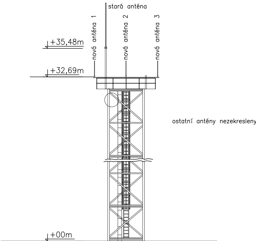
Pohled na příhradový stožár VHF vysílací středisko Kopec Písek 1:200
