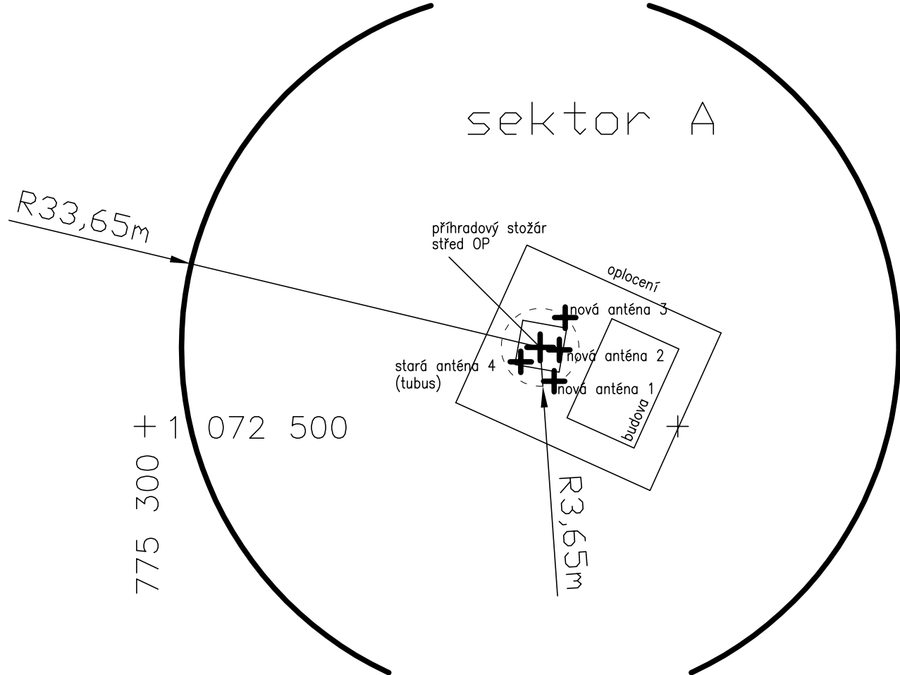
Pohled na příhradový stožár VHF vysílací středisko Kopec Písek 1:200
