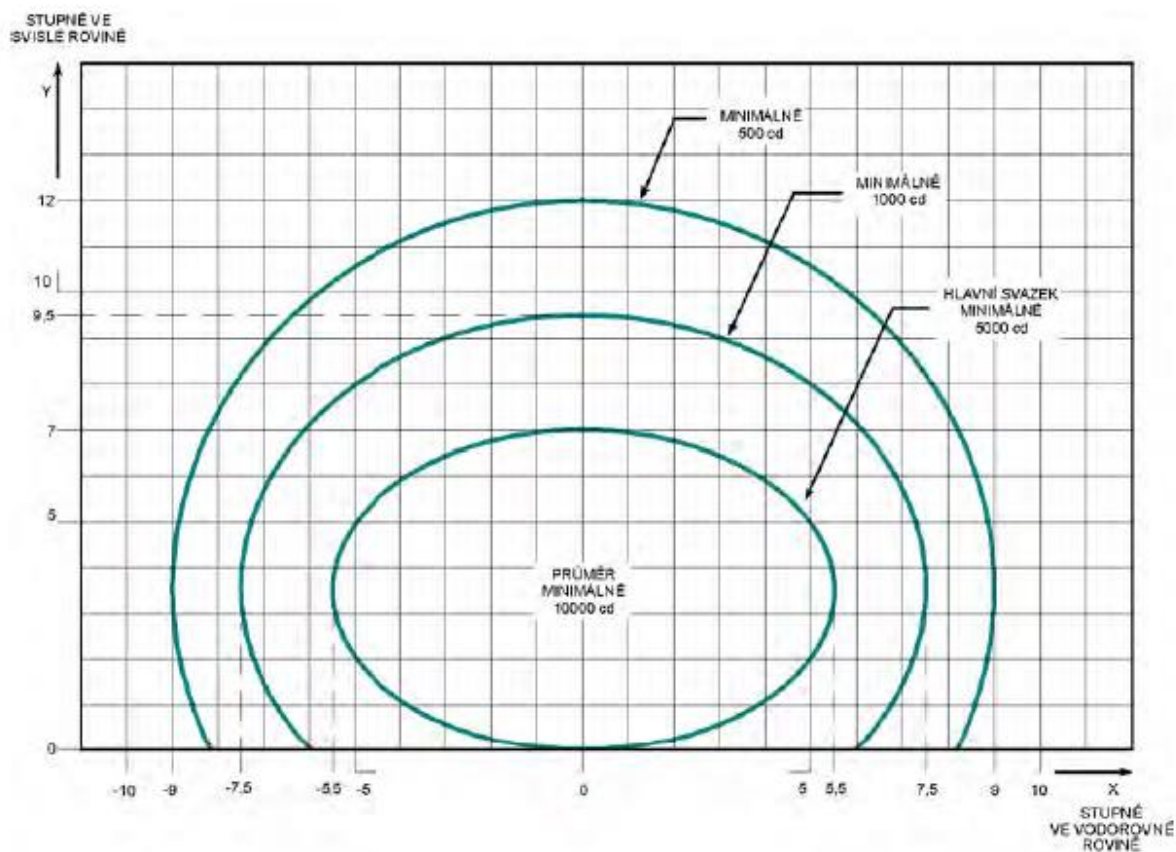
Obrázek U-13. Izokandelový diagram pro postranní dráhová návěstidla, kde je šířka RWY 45 m (bílá návěstidla)
