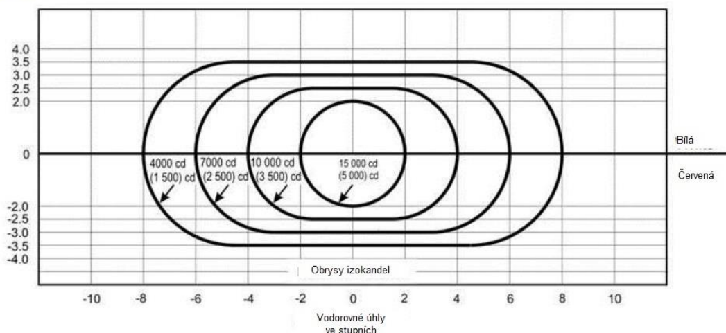
Obrázek U-26. Rozložení svítivosti soustav PAPI a APAPI
