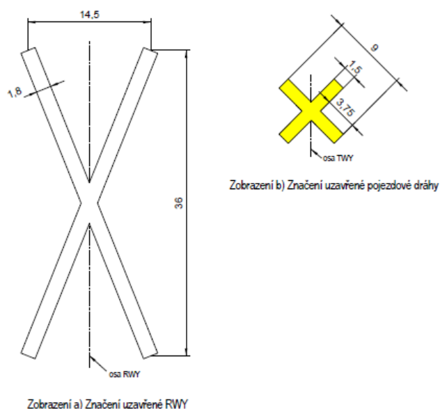
Obrázek R-1. Značení uzavření RWY a pojezdové dráhy
