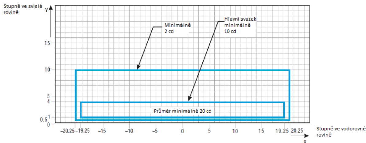
Obrázek U-20. Izokandelový diagram pro osová návěstidla pojezdové dráhy (rozestup 7,5m, 15 m a 30 m), příček zákazu vstupu a stop příček v obloucích zatáček určený pro použití v podmínkách RVR 350 m a více
