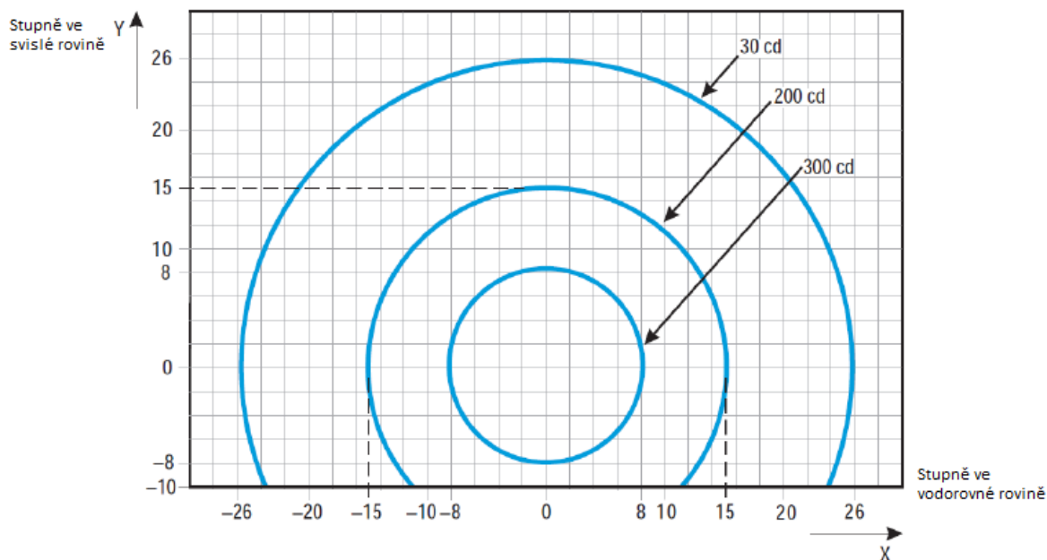
Obrázek U-27. Izokandelový diagram pro každé z dráhových ochranných návěstidel nízké svítivosti, v uspořádání typu A
