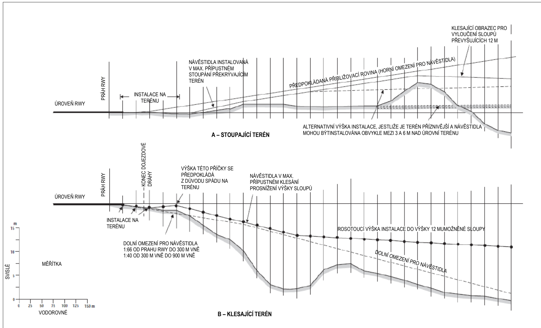
Obrázek GM-M-1. Svislé tolerance instalace
