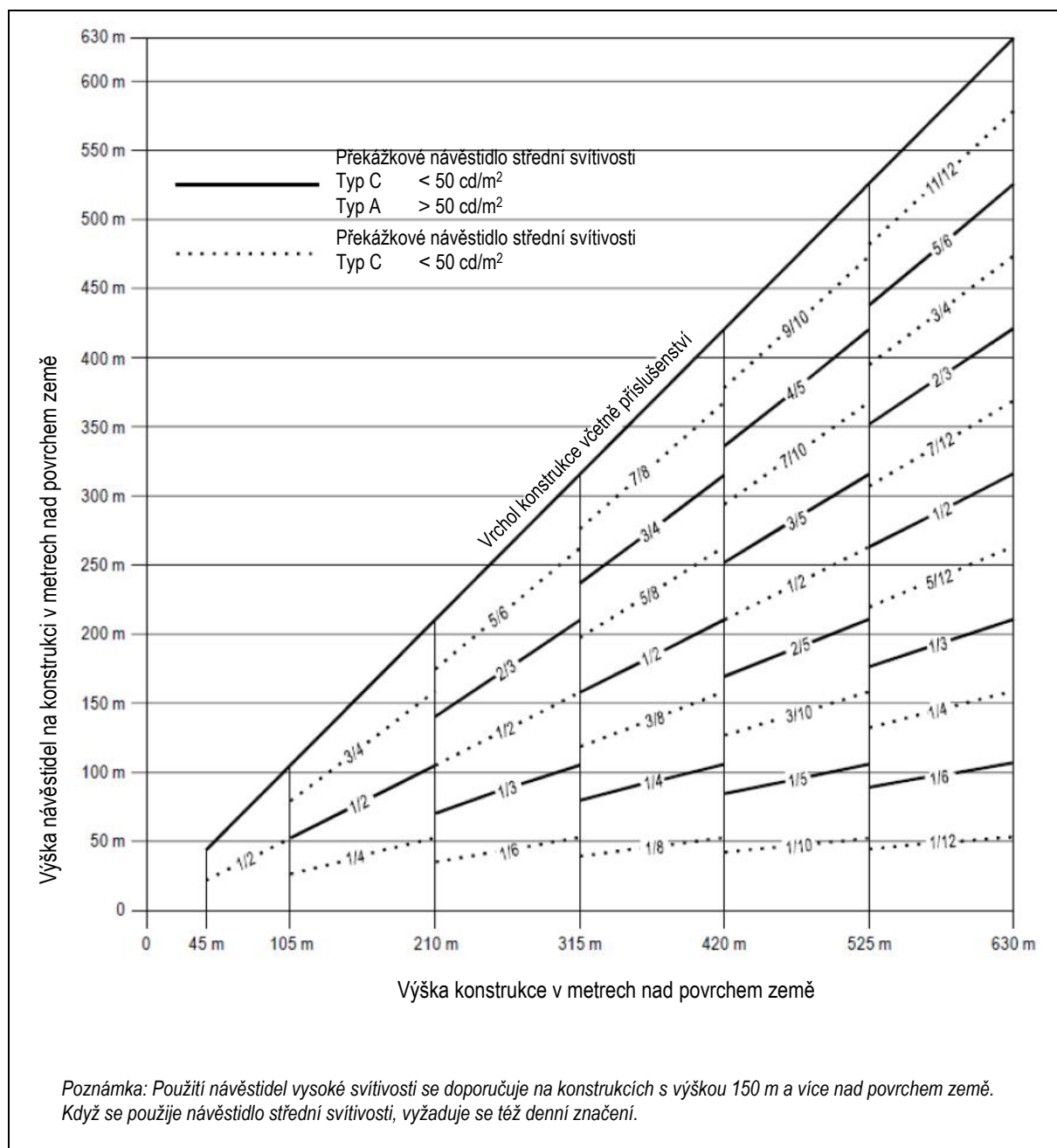
Obrázek GM-Q-5. Duální systém překážkových návestidel střední svítivosti typu A/typu C
