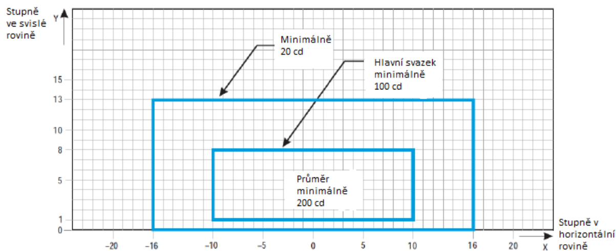
Obr. U-16. Izokandelový diagram pro osová návěstidla pojezdové dráhy (rozestup 15 m), návěstidla REL, příček zákazu vstupu a stop příček v přímých částech určený pro použití v podmínkách RVR nižší než o hodnotě 300 m, kde se mohou vyskytnout velká překrytí a pro dráhová ochranná návěstidla nízké svítivosti v uspořádání typu B
