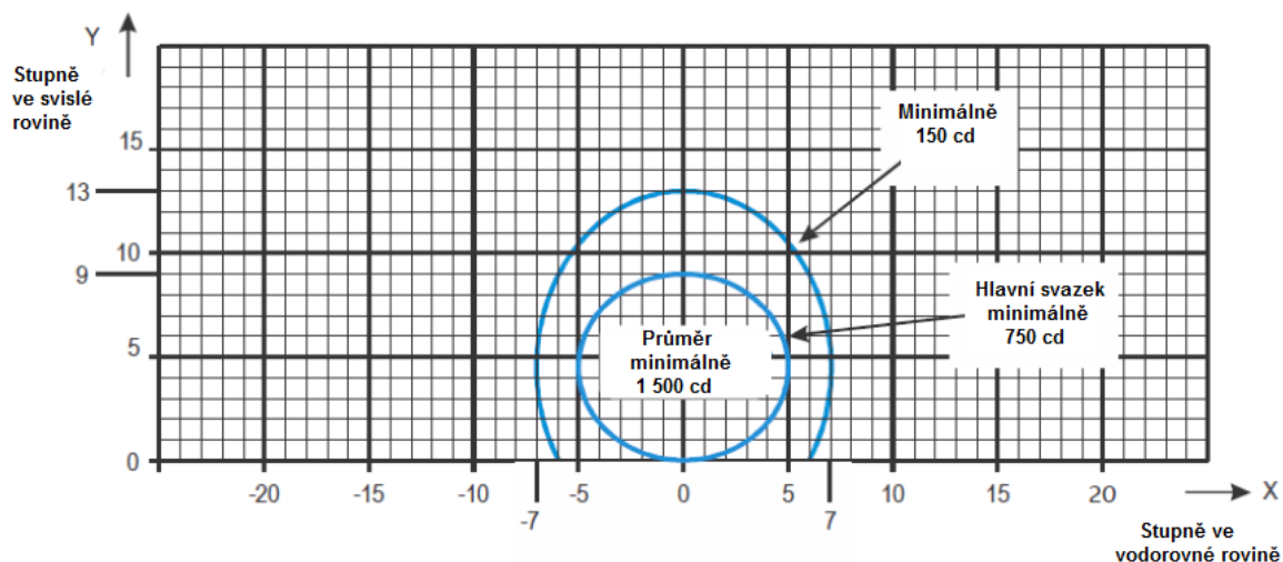
Obrázek U-29. Izokandelový diagram vyčkávacích návěstidel pro vzlet (THL) (červené návěstidlo)
