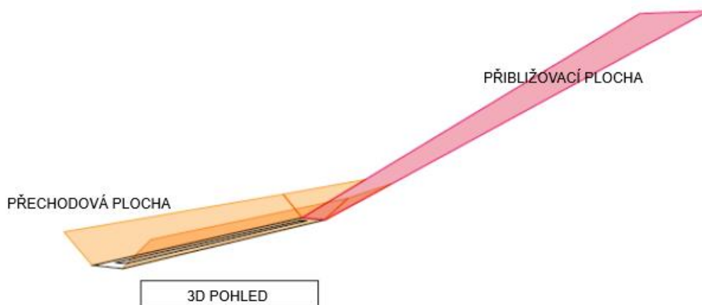
Obrázek 4-1. Přibližovací plocha a přechodová plocha
