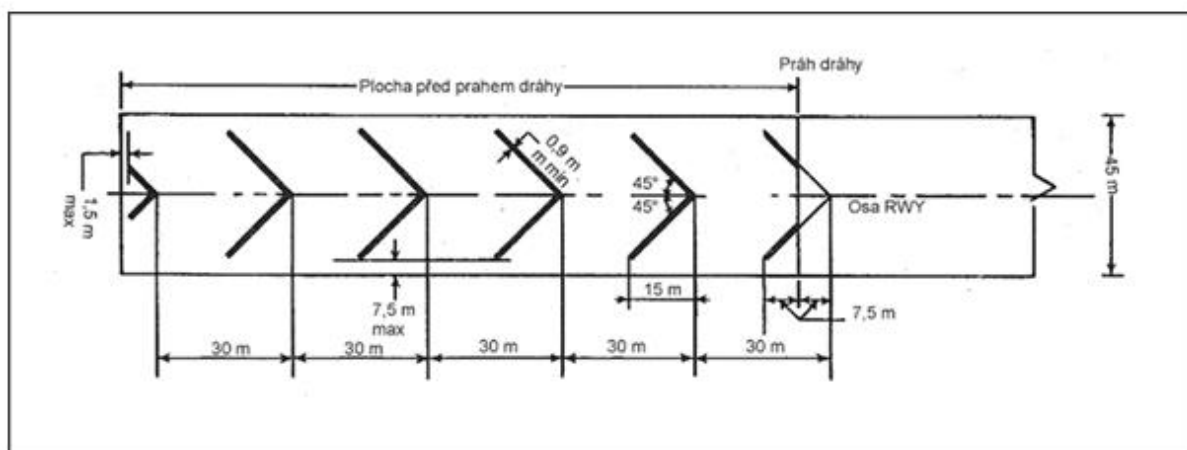
Obr. 7-3. Značení před prahem dráhy
