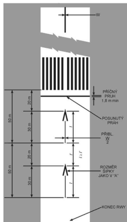
B. Trvale posunutý práh dráhy
