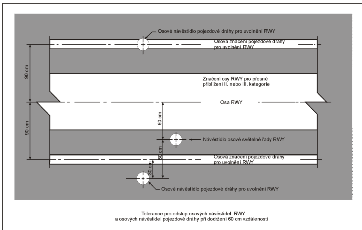
Obr. 5--273. —Odstup osových návěstidel RWY a pojezdové dráhy
