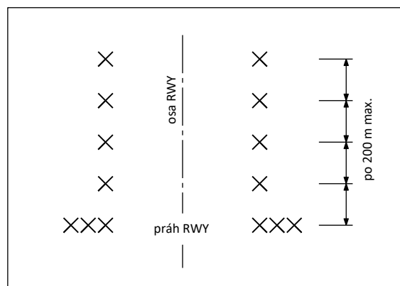
Obr. 5-330A. —Značky zasněžených RWY
