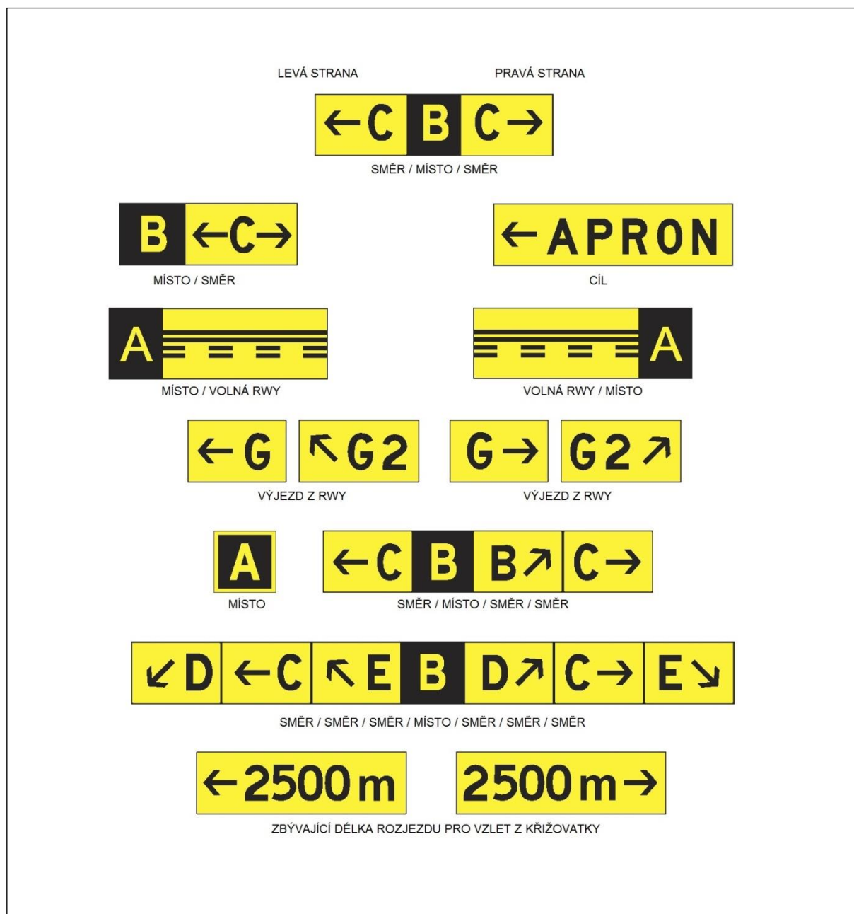
Obr. 5-2831. — Informační znaky
