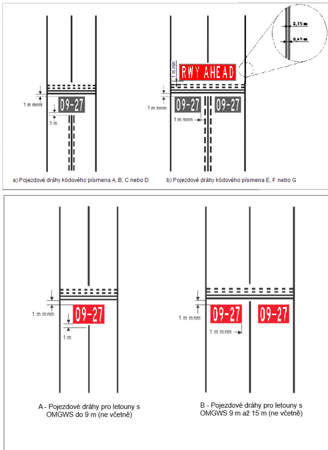
Obr. 5-10. — Příkazové značení, výstražné značení a postranní značení pojezdové dráhy
