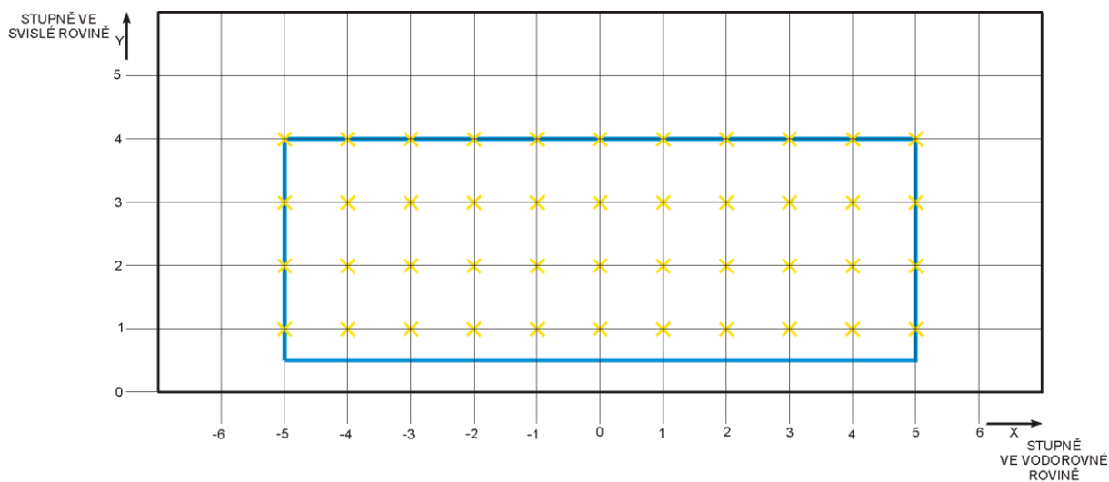
Obr. 2.21 – Bodová síť, která se užívá pro výpočet průměrné svítivosti osových návěstidel pojezdové dráhy a stop příček
