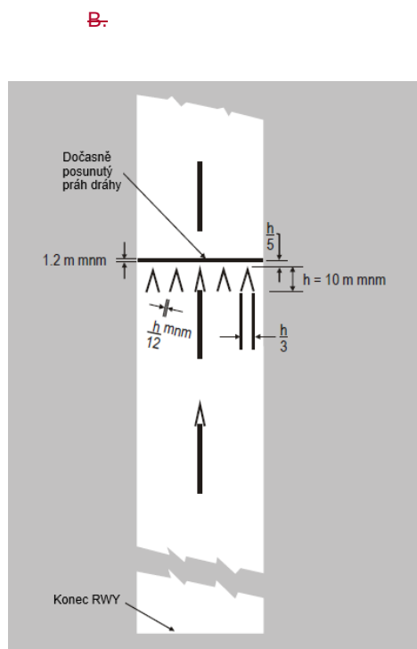
A. Dočasně posunutý práh dráhy
