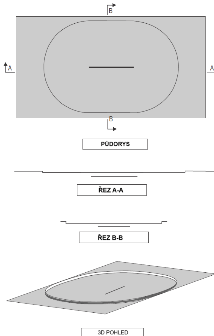
Obrázek 4-5. Plocha pro přímé přiblížení podle přístrojů
