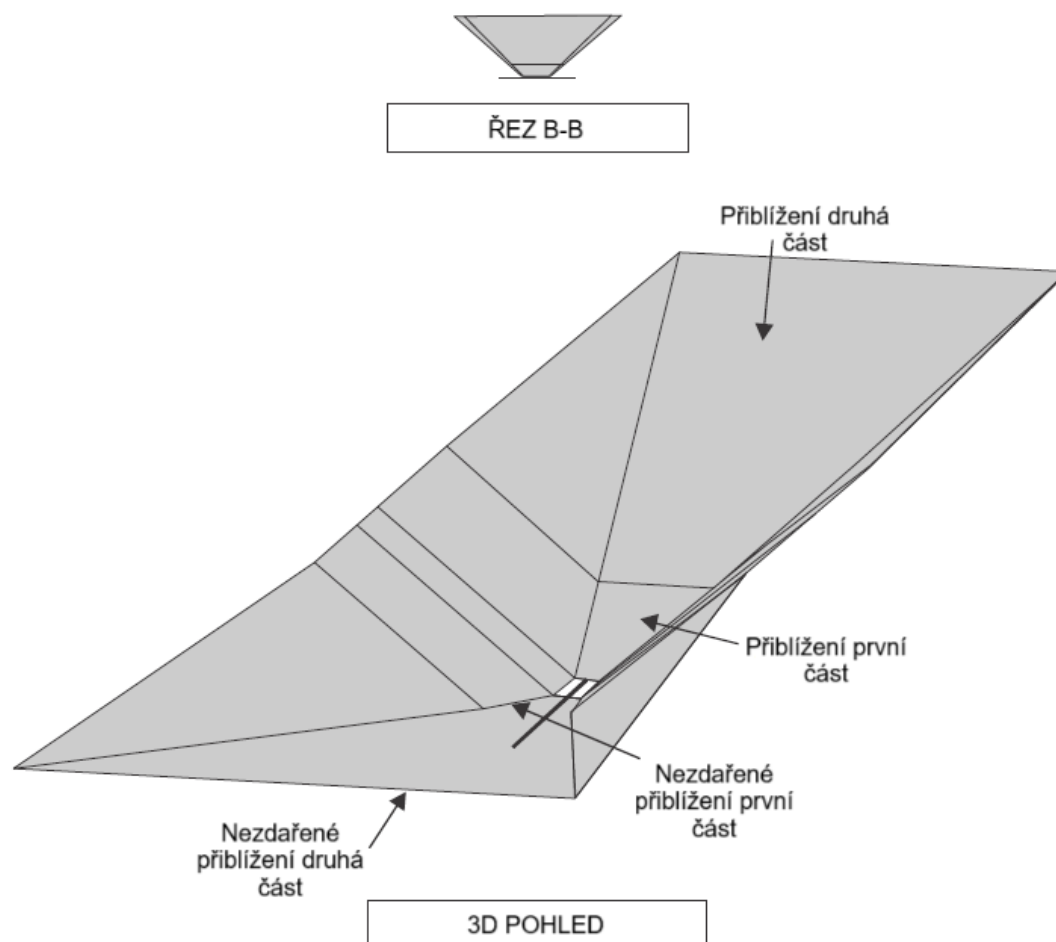
Obrázek 4-6. Plocha pro přesná přiblížení
