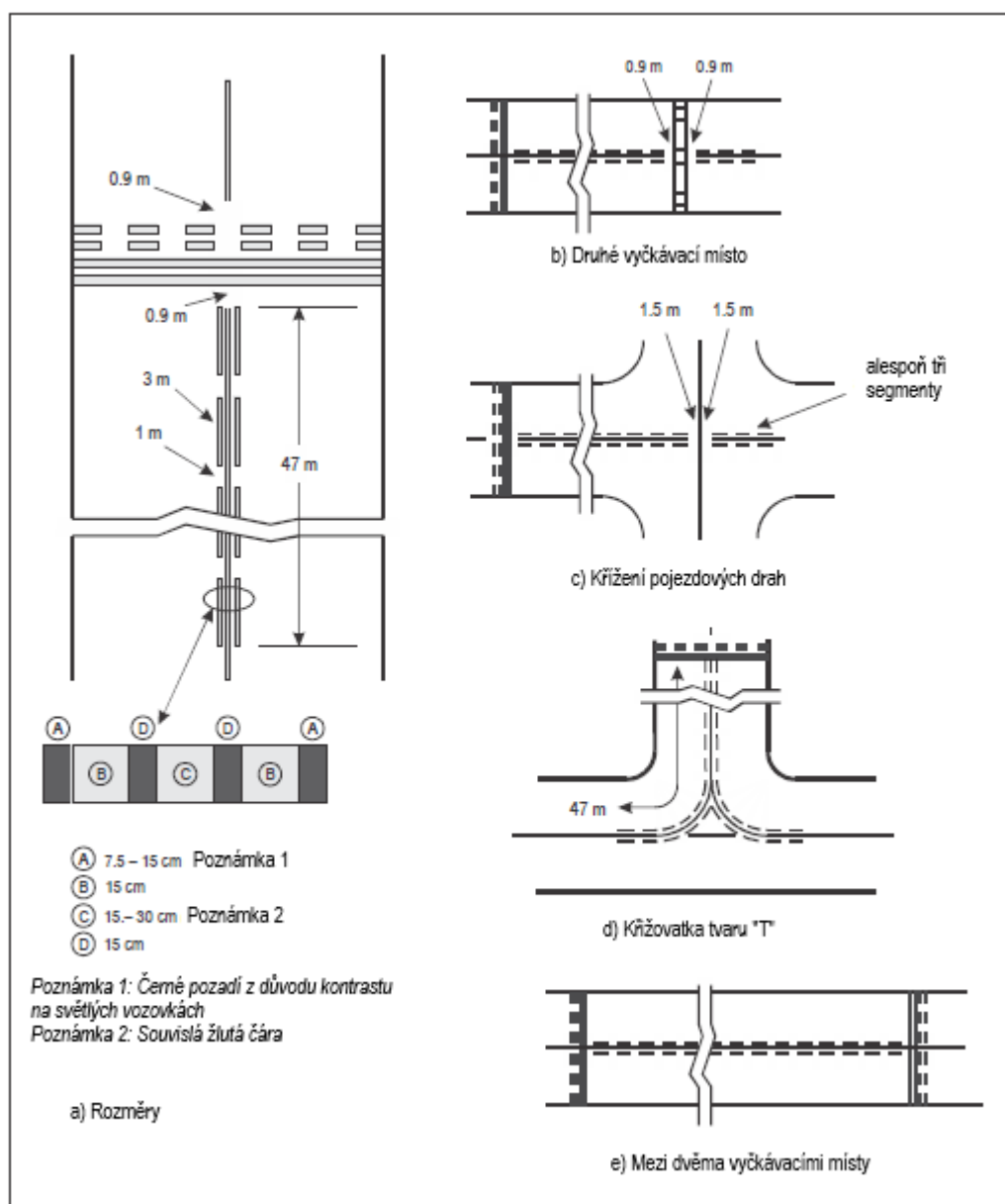
Obr. 5-7. — Zvýrazněné značení osy pojezdové dráhy
