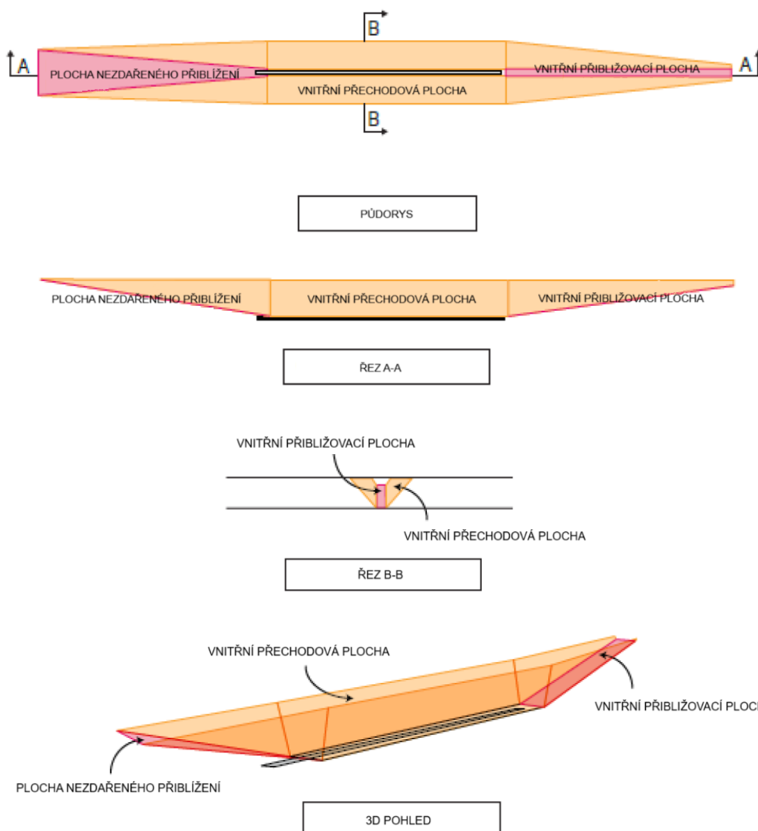
Obrázek 4-3. Bezpřekážkový prostor na RWY pro přesné přiblížení
