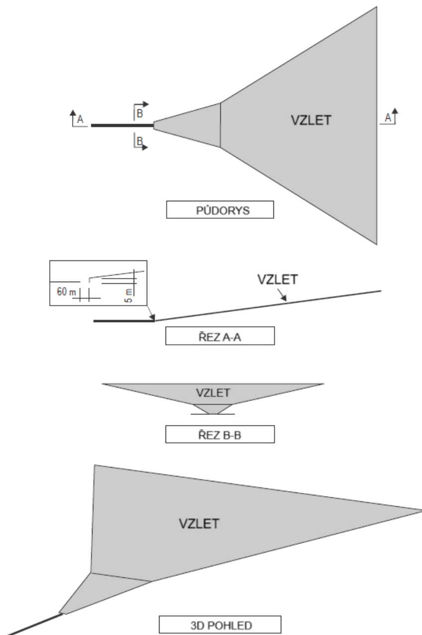
Obrázek 4-7. Plocha pro přístrojový odlet
