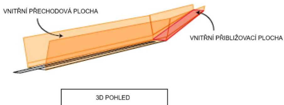
Obrázek 4-2. Vnitřní přibližovací a přechodové plochy na RWY pro nepřesné přístrojové přiblížení
