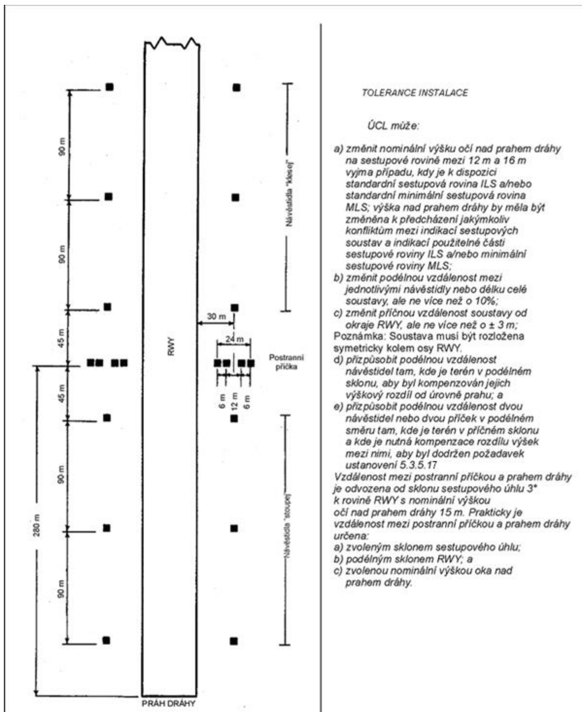
Obr. 5-174. Umístění návěstidel pro T-VASIS
