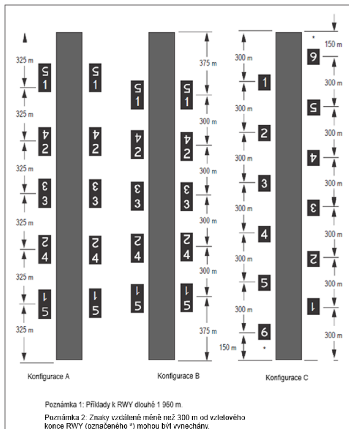
Obr. A-10 Konfigurace RDRS
