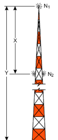
Obr. 6-2a. — Příklad značení a světelného označení vysokých konstrukcí
