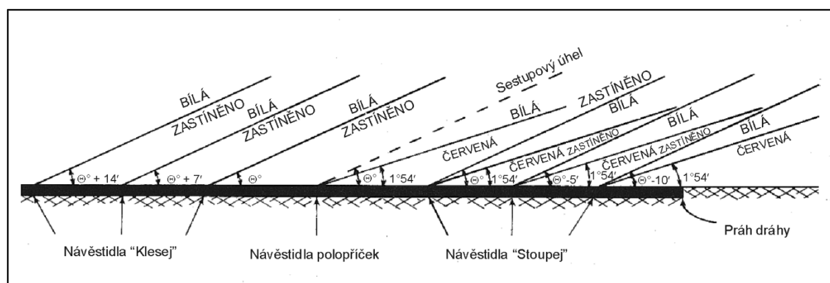
Obr. 5—18.5 —Světelné svazky a úhly náměru T-VASIS a AT-VASIS
