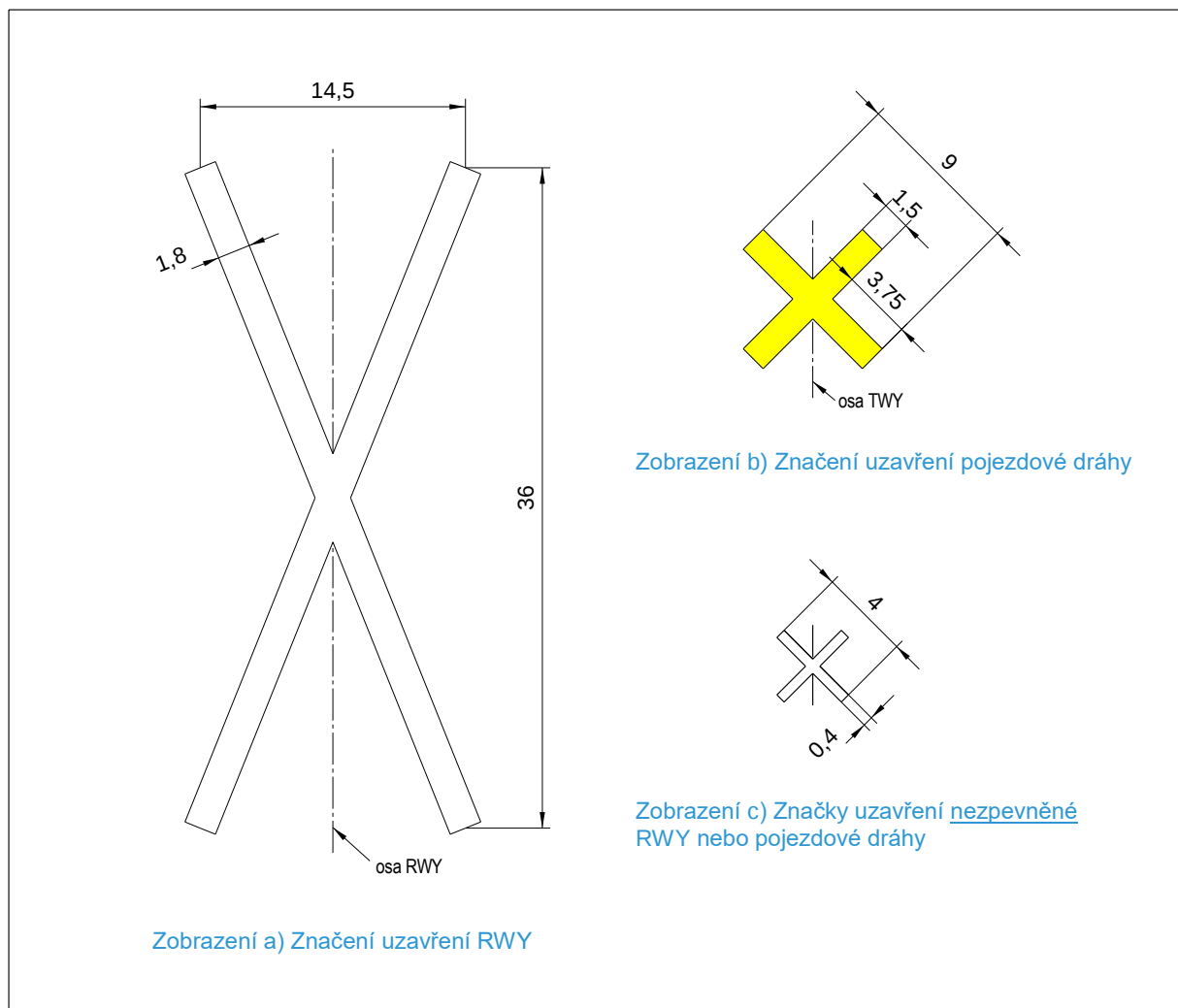
Obr. 7-1. — Značení, značky uzavření RWY a TWY[ŠH1]
