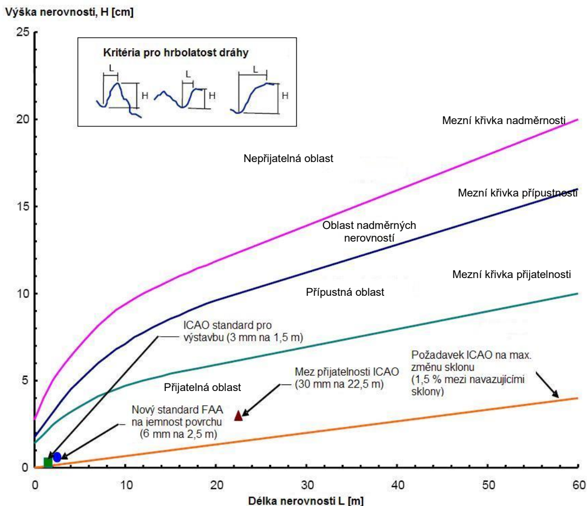
Obr. A-2A3. — Porovnání kritérií na hrboлатost povrchu
