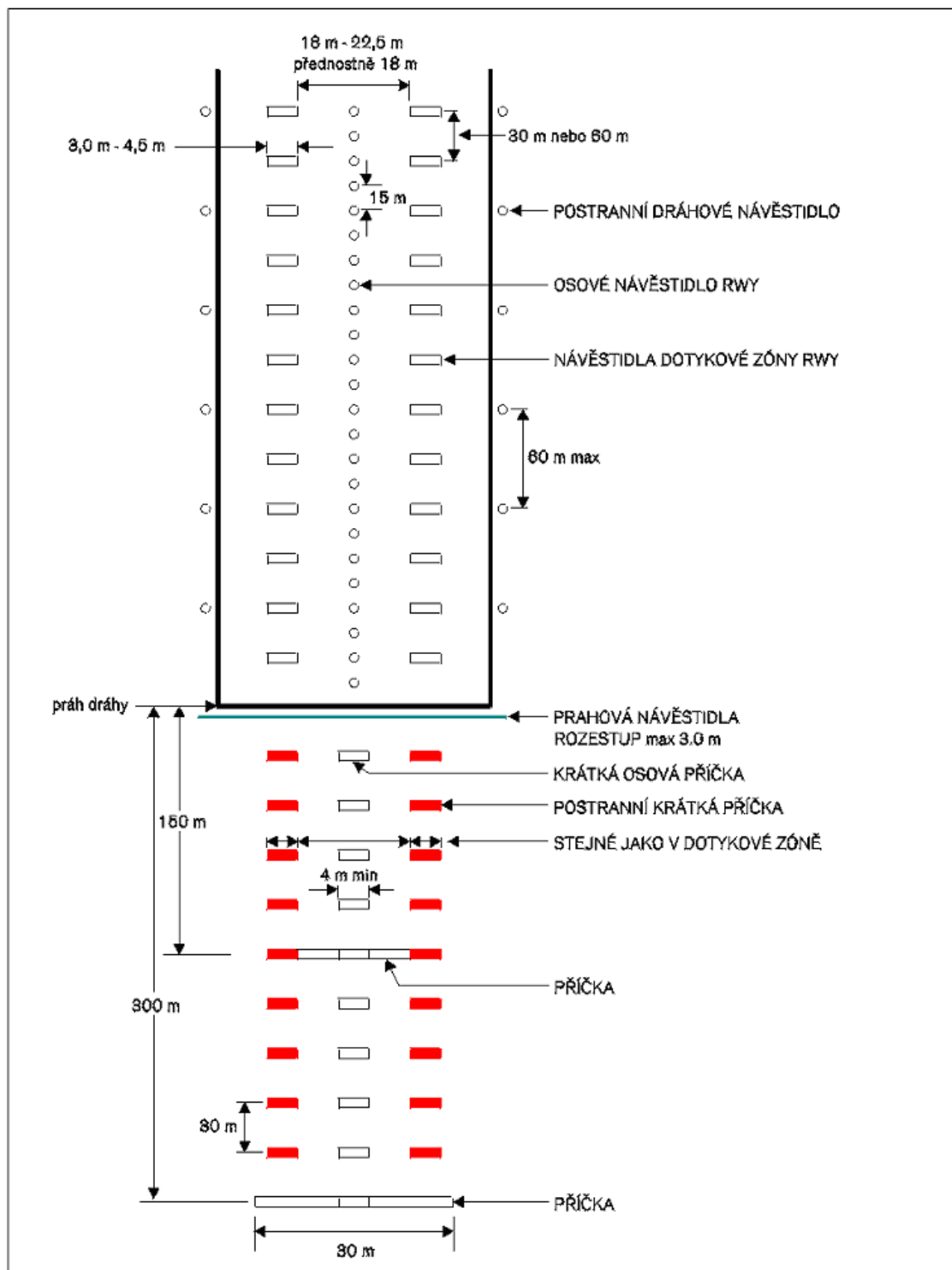
Obr. 5-141. — Vnitřních 300 m světelné přiblížovací a dráhové soustavy pro RWY pro přesné přiblížení II. a III. kategorie
