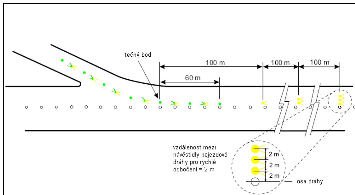
Obr. 5-25. Návěstidla pojezdové dráhy pro rychlé odbočení
