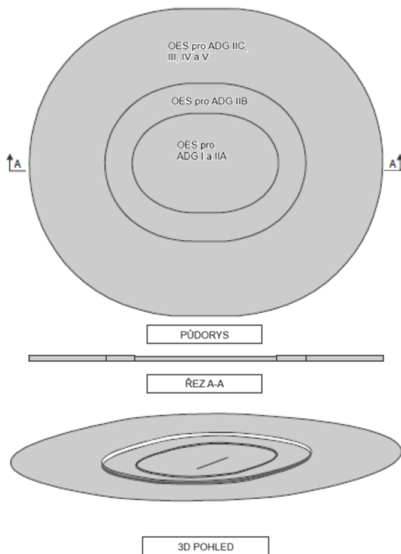
Obrázek 4-4. Vodorovná plocha
