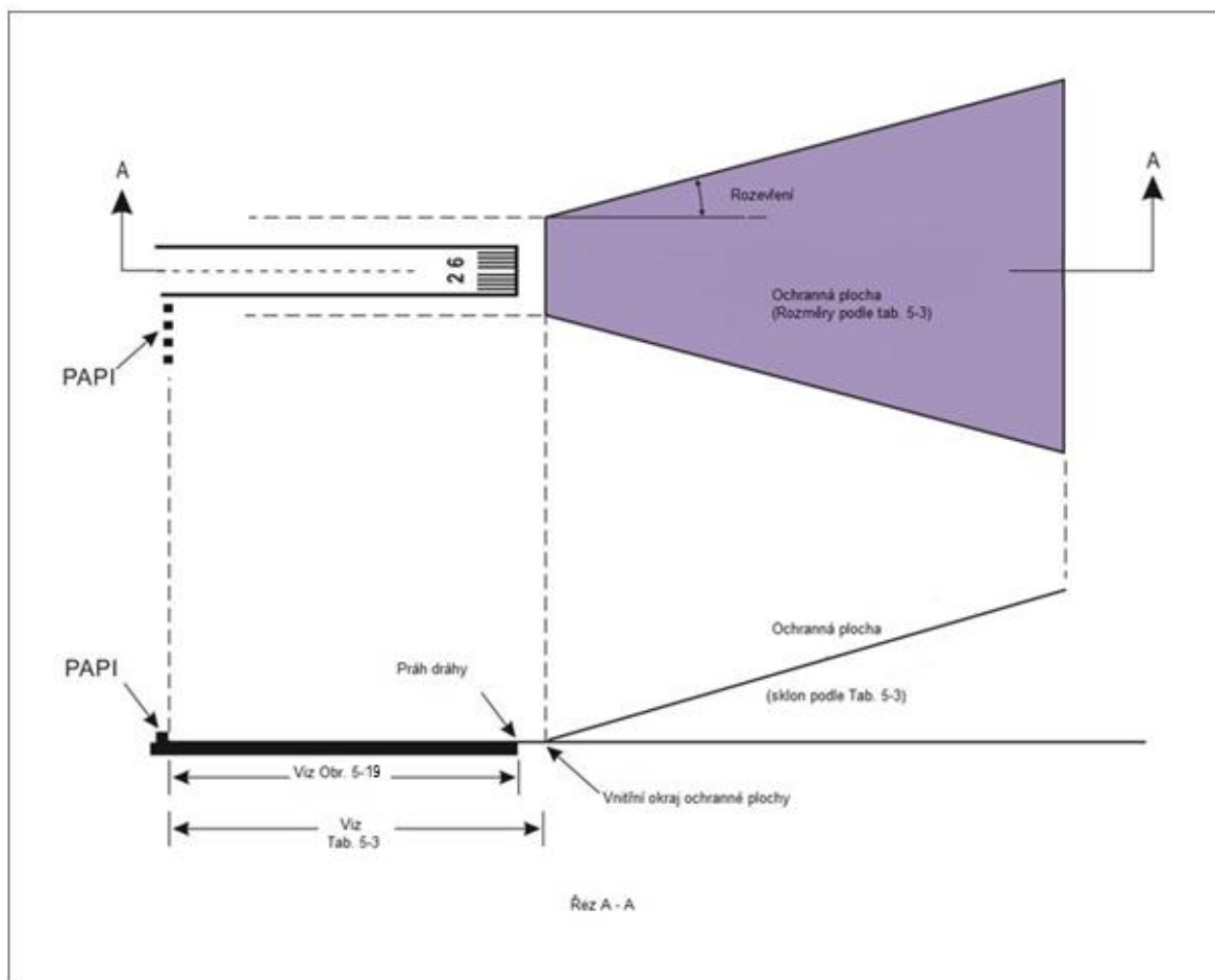
Obr. 5-1821. Ochranná plocha pro světelné sestupové soustavy pro vizuální přiblížení
