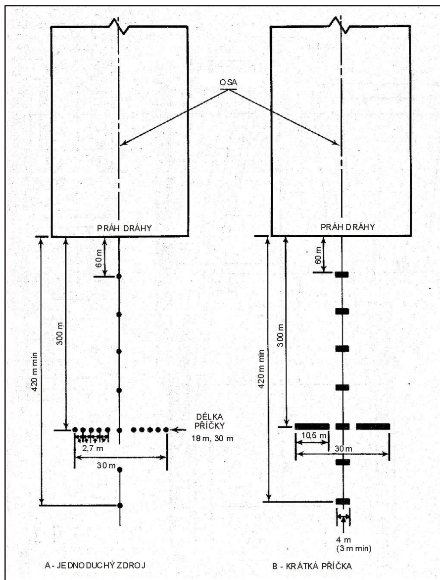
Obr. A-76 Jednoduché přibližovací světelné soustavy
