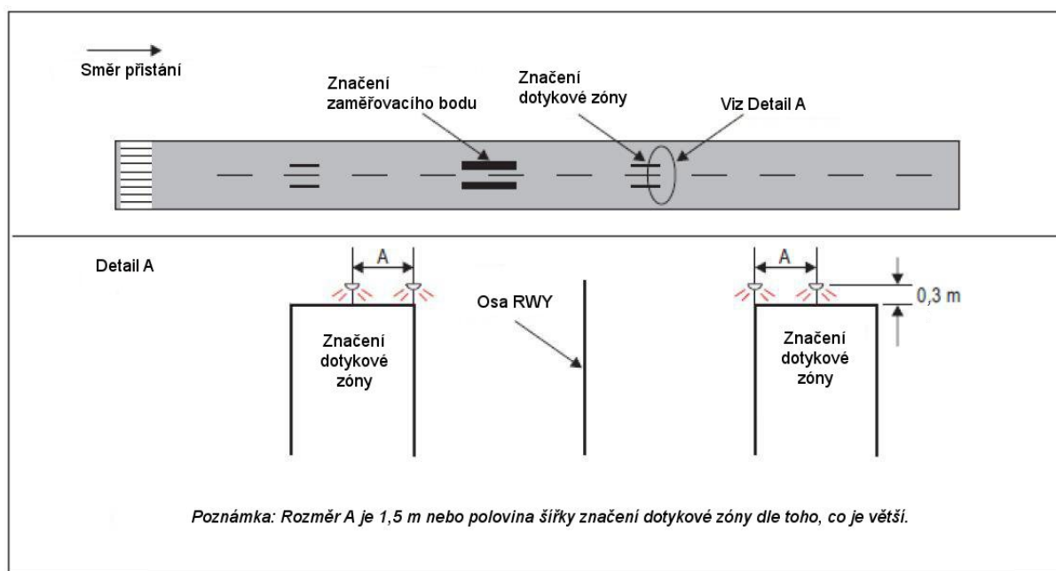
Obr. 5-24. — Jednoduchá návěstidla dotykové zóny
