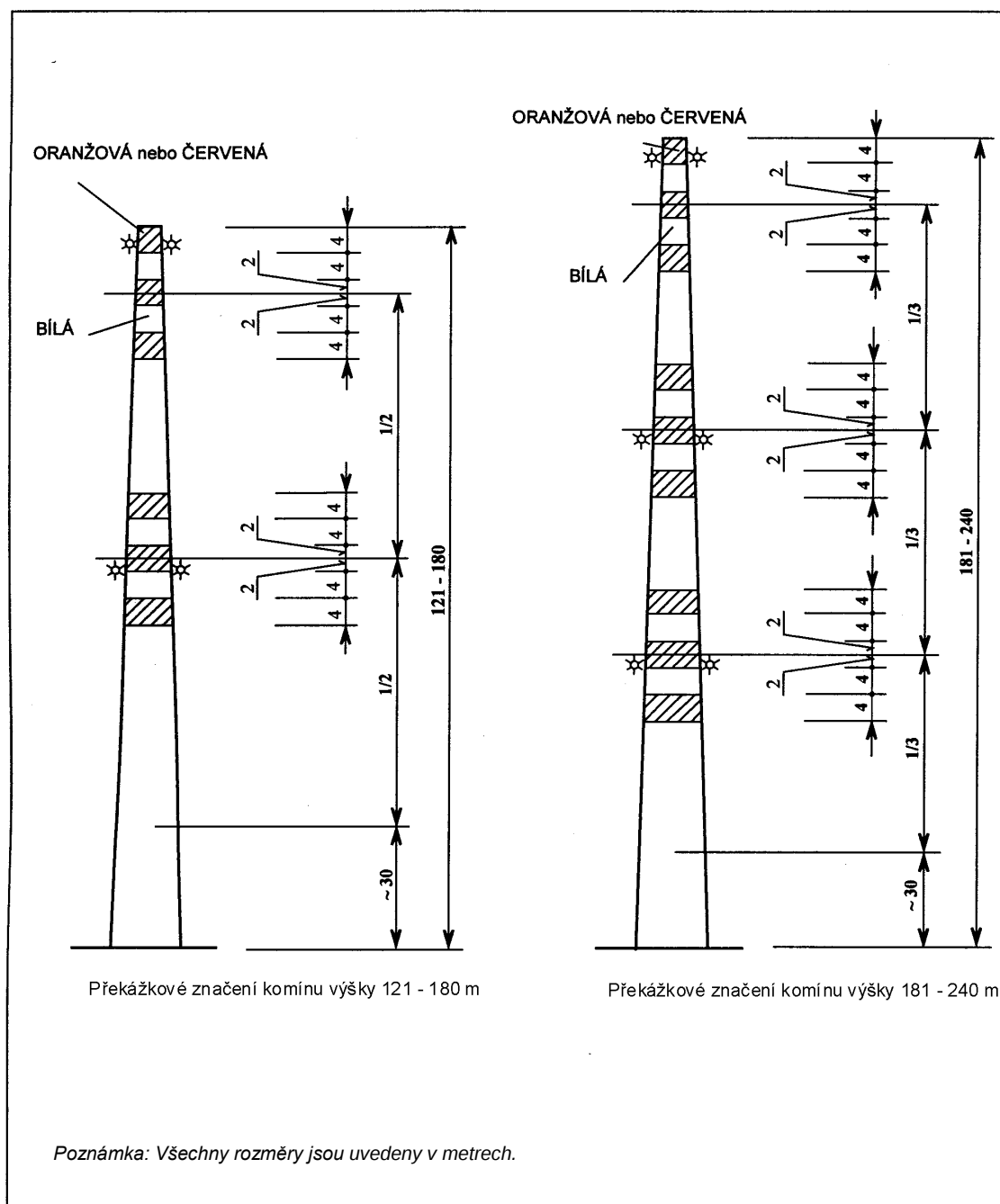
Obr. 6-2c. Překážkové značení komínu nad 120 m
