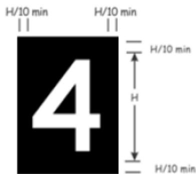
Obr. 4.5 Rozměry znaku RDRS
