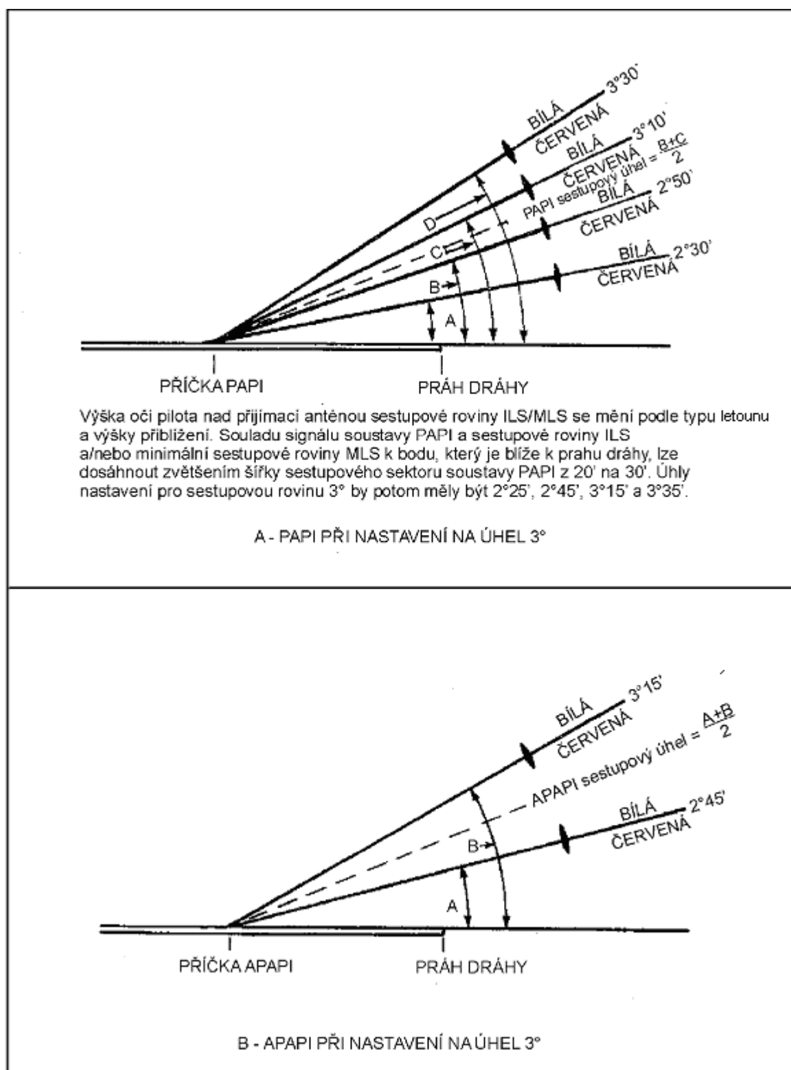
Obr. 5-2017. Světelné paprsky a úhel výškového nastavení soustavy PAPI a APAPI
