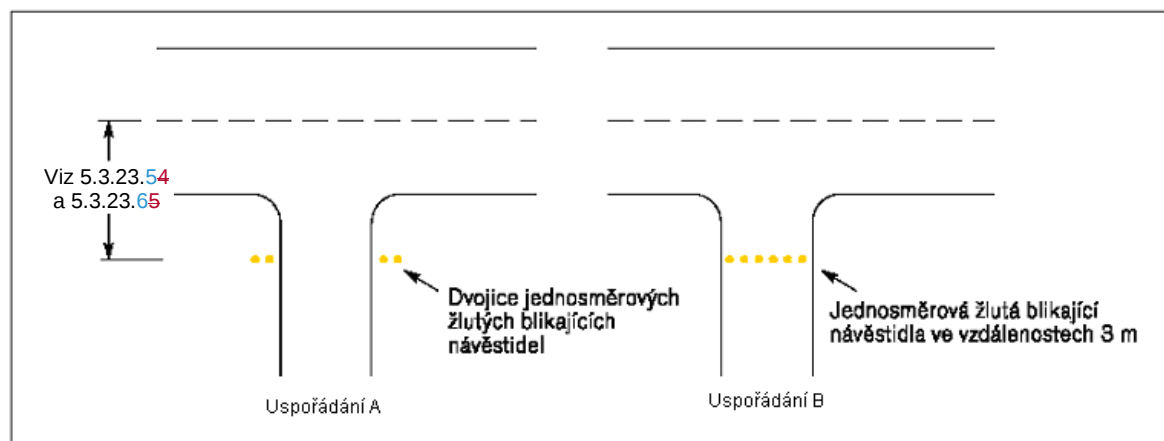
Obr. 5--296. —Dráhová ochranná návěstidla
