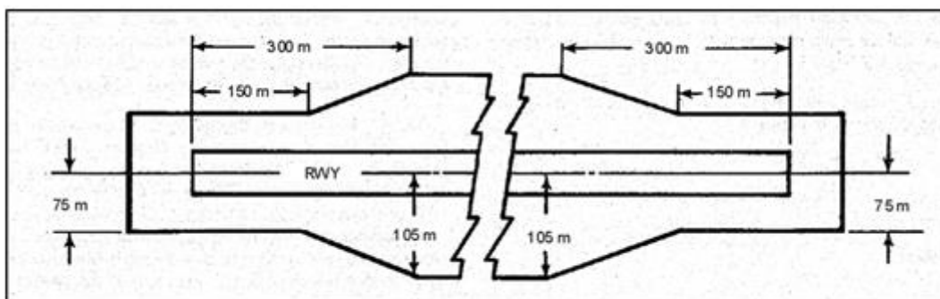
Obr. A-4 Upravená část vzletového a přistávacího pásu zahrnujícího RWY pro přesné přiblížení kódového čísla 3 nebo 4
