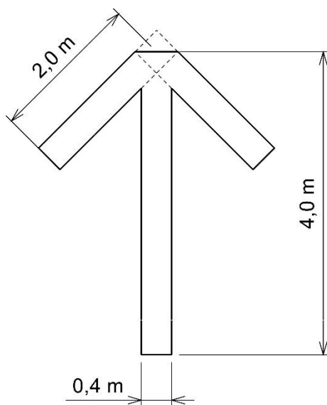
Obr. 5--34A2. Značka přistání kluzáků
