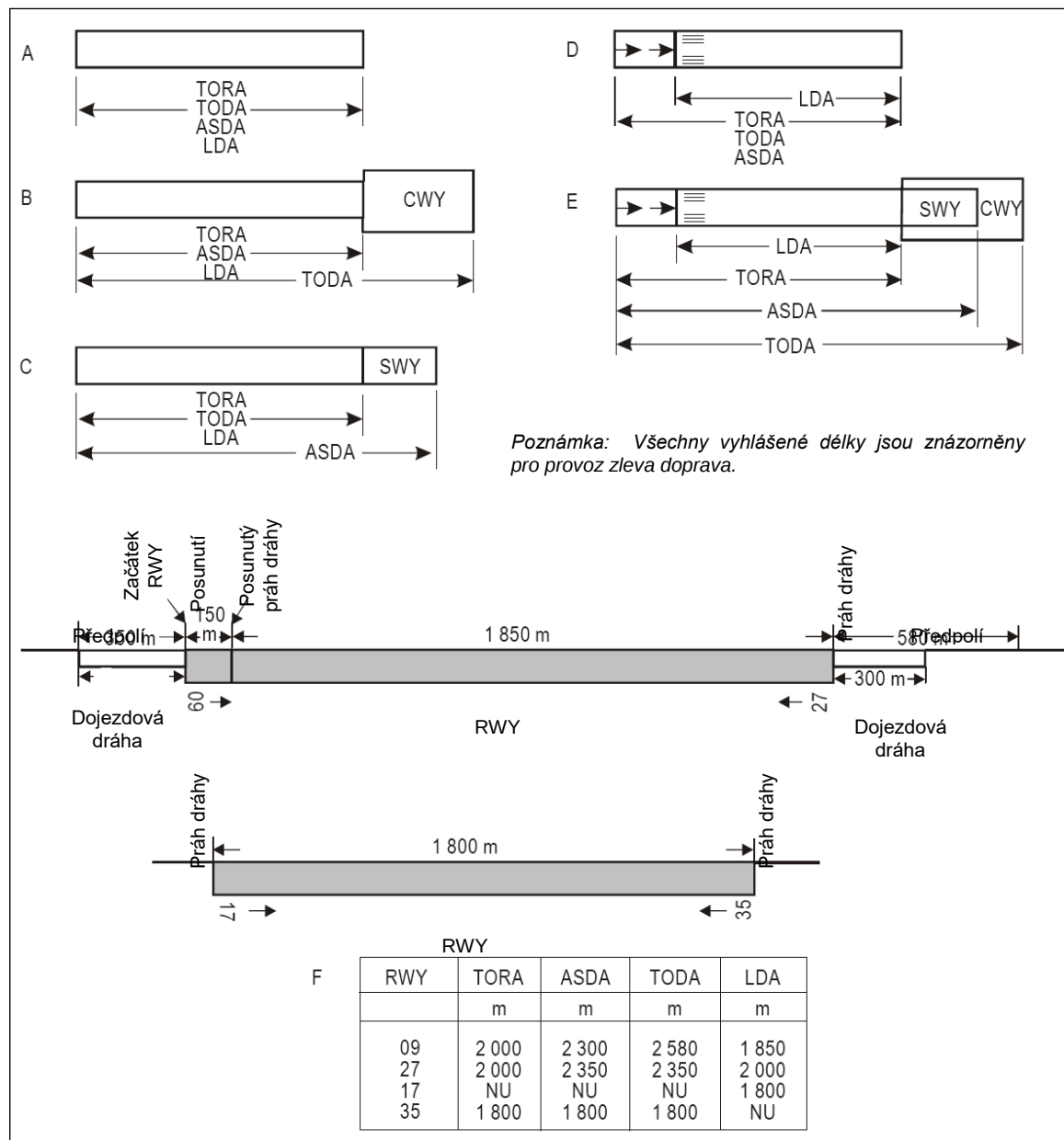
Obr. A-1. Znázornění vyhlášených délek
