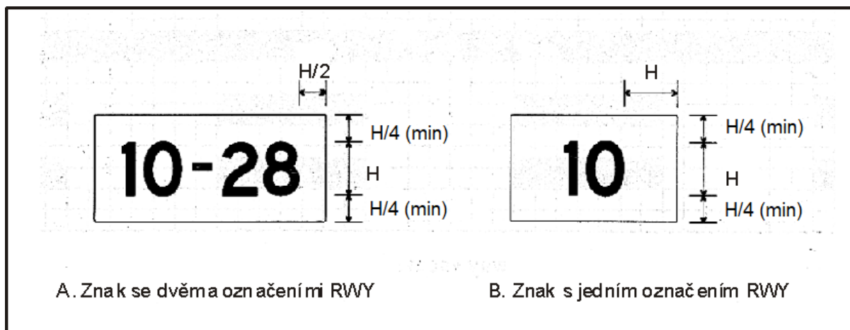
Obr. 4.4 Rozměry znaků
