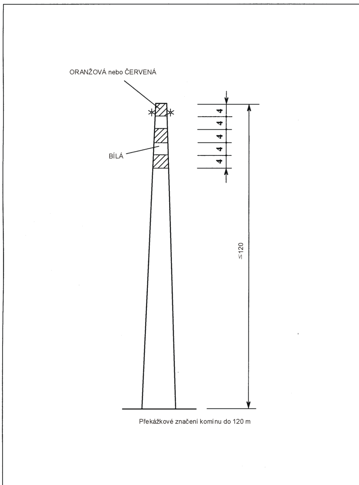
Obr. 6-2b. Překážkové značení komínu do 120 m
