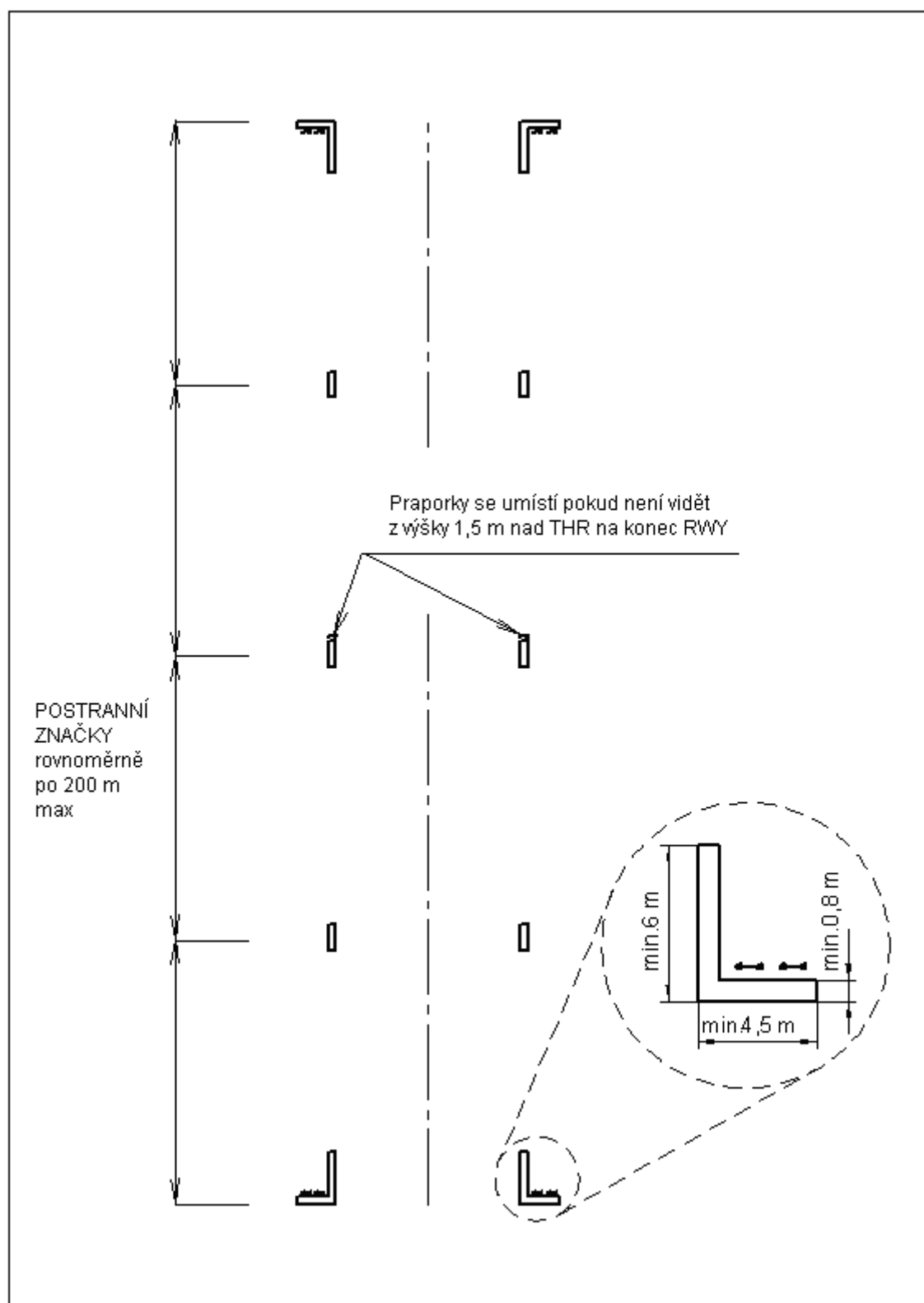
Obr. 5-2-2b. —Postranní dráhové značky, prahové značky dráhy
