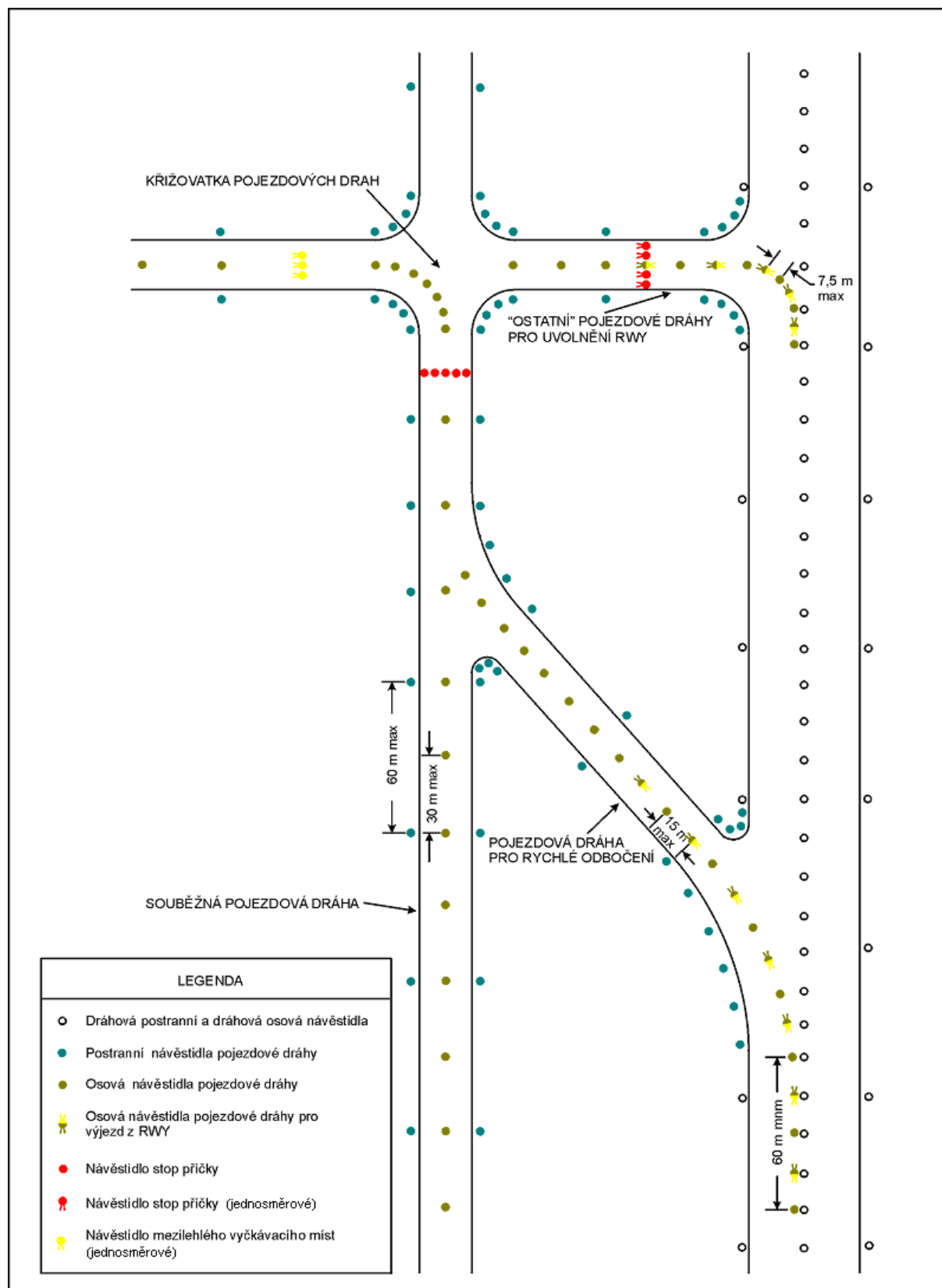
Obr. 5--262. -Návěstidla na pojezdové dráze
