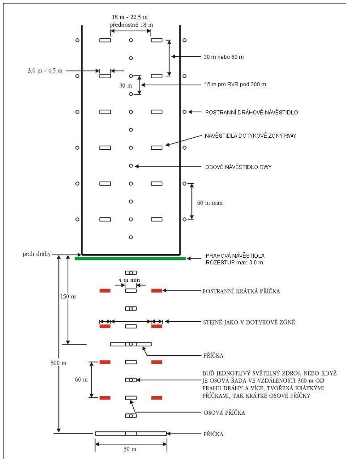
Obr. 5-152. — Vnitřních 300 m světelné přibližovací a dráhové soustavy pro RWY pro přesné přiblížení II. a III. kategorie, když může být prokázána úroveň údržby návěstidel splňující požadavky Hlavy 10.
