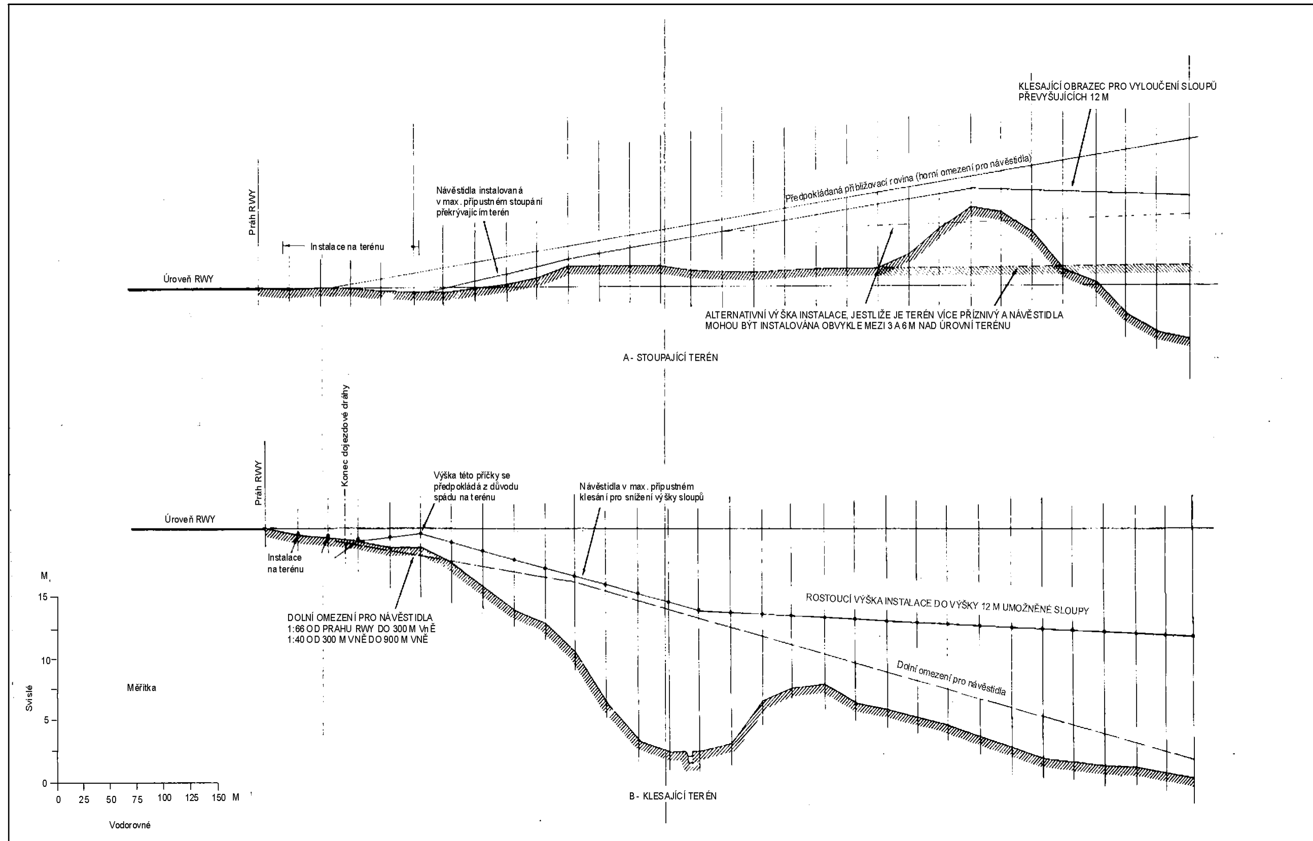
Obr. A-98. — Svislé tolerance instalace
