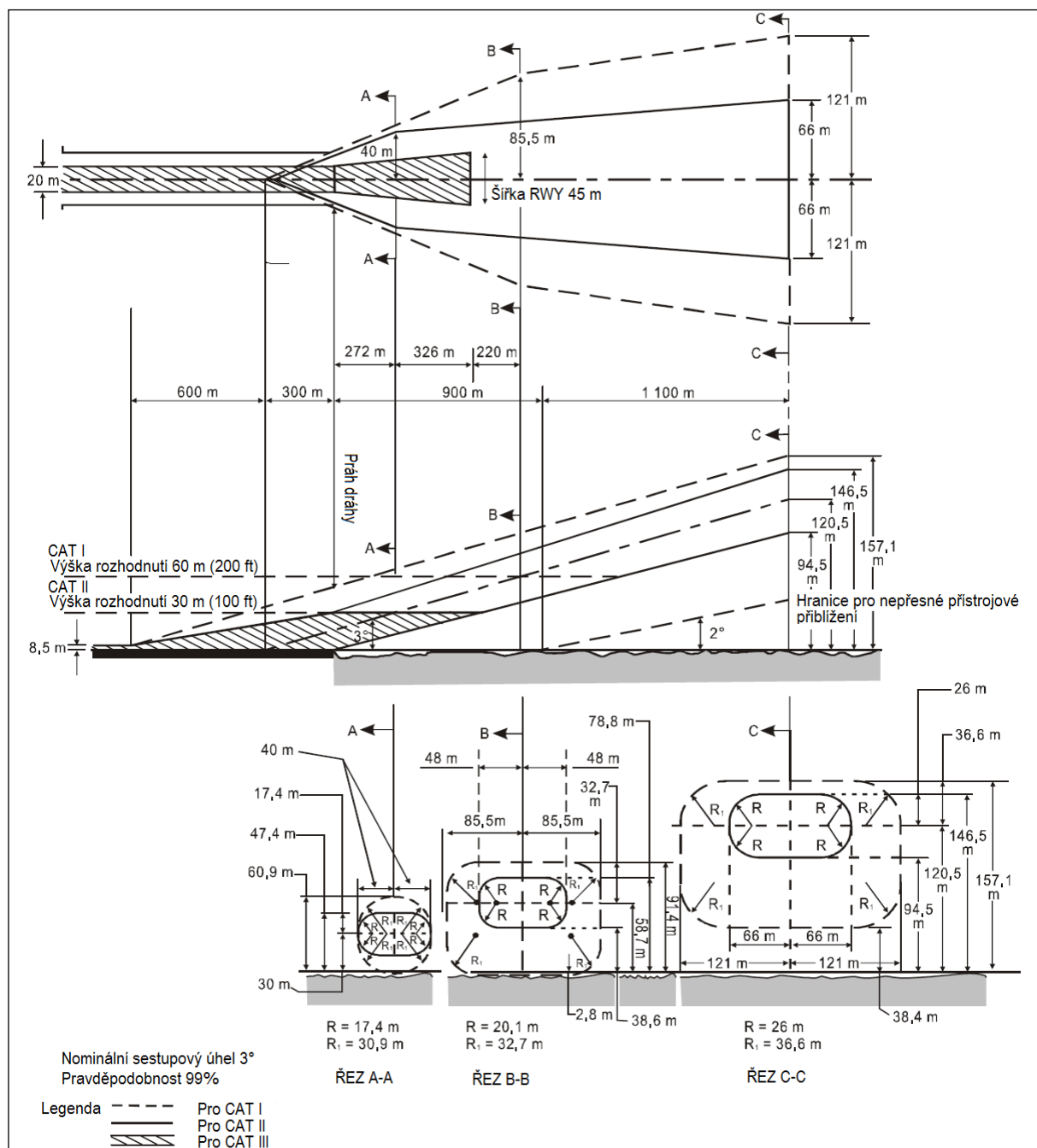
Obr. A-6 Obálky sestupové dráhy pro navrhování přibližovací světelné soustavy pro přesné přiblížení CAT I. II a III
