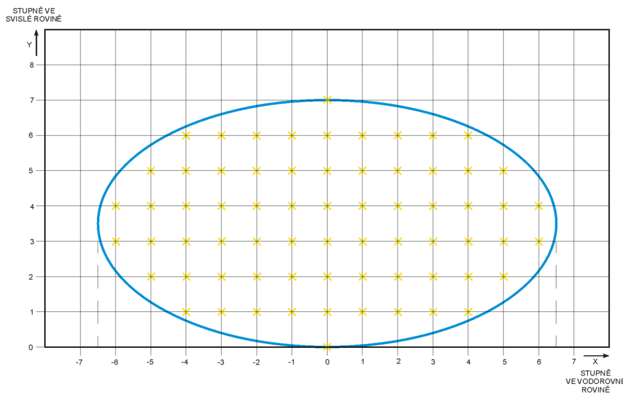
Obr. 2.11 – Bodová síť používaná pro výpočet průměrné intenzity přibližovacích a dráhových návěstidel
