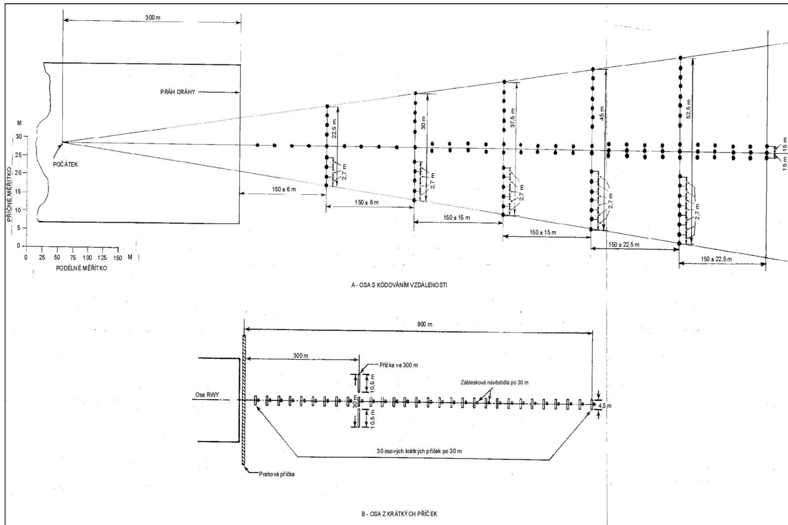
Obr. A-87. — Přibližovací světelné soustavy pro přesné přiblížení I. kategorie
