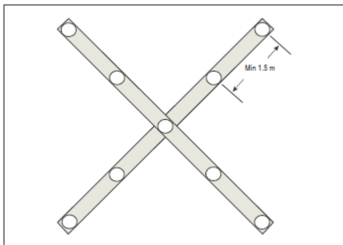
Obr. 7-2. Příklad návěstidel uzavření RWY s pěti návěstidly na rameni v odpovídající svislé poloze
