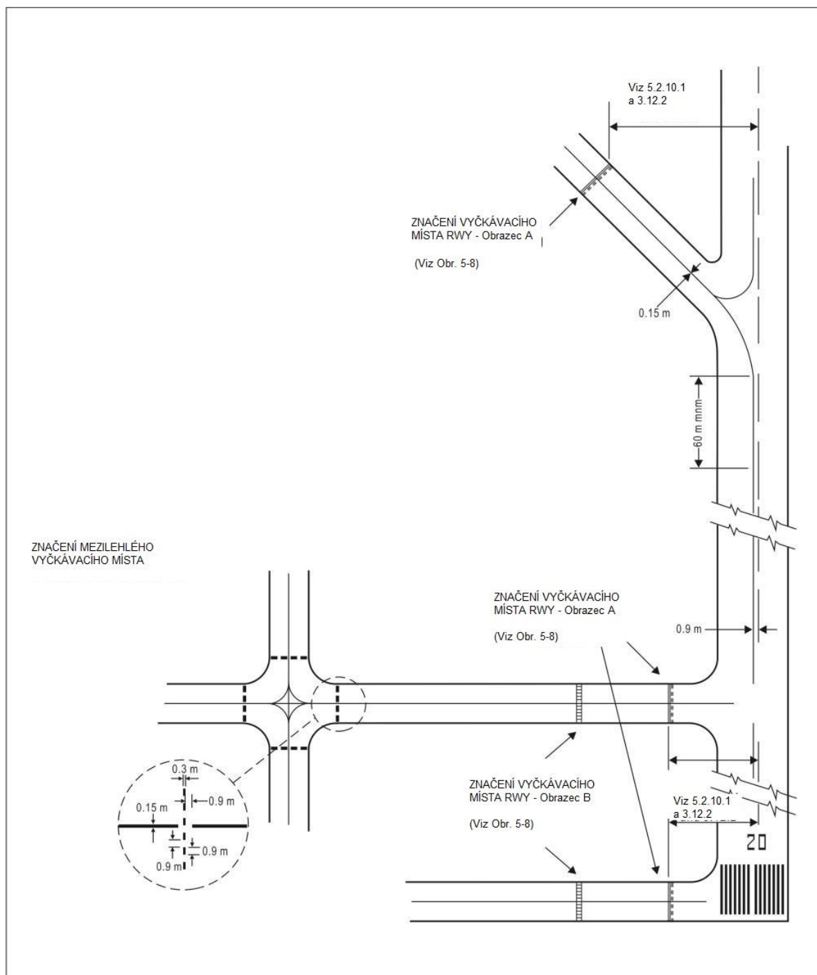
Obr. 5-6. — Značení na jezdové dráze
