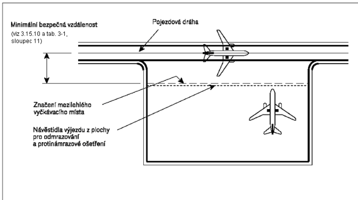
Obr. 5--285. —Typická vzdálená plocha pro odmrazování a protinámrazové ošetření
