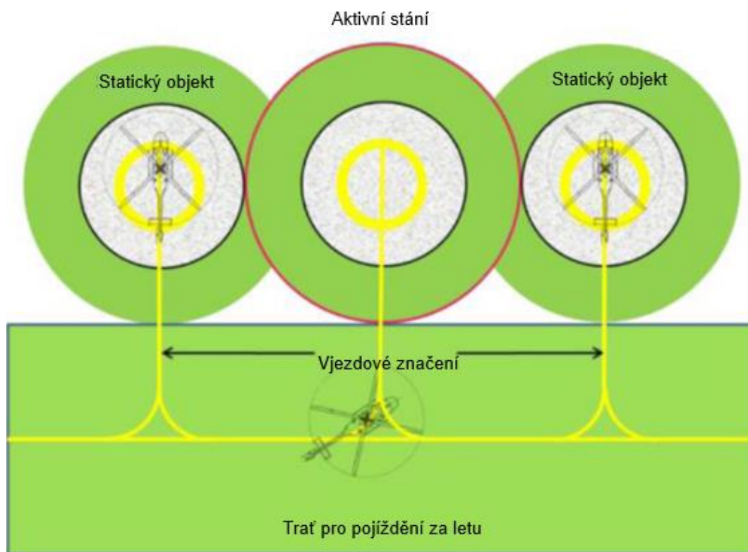
Obr. 3-9 Stání pro otáčení (s tratí pro poježdění za letu) nesouběžné použití – aktivní vnitřní stání
