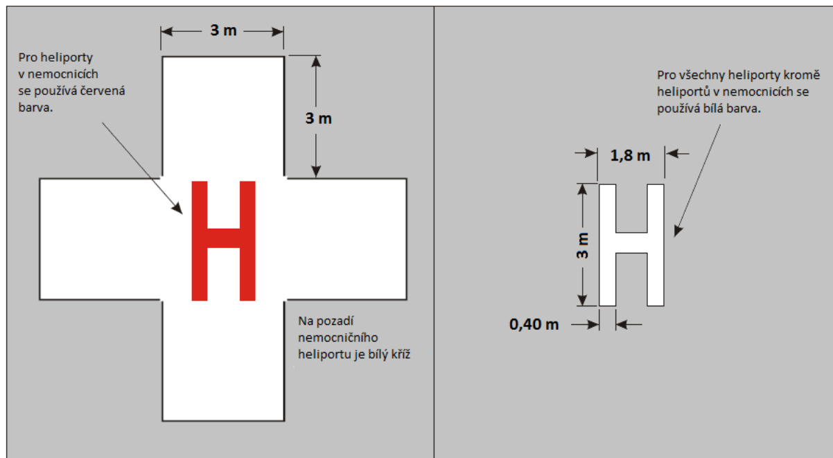
Obr. 5-42 Poznávací značení heliportů v nemocnicích/pro leteckou záchrannou a poznávací značení ostatních heliportů
