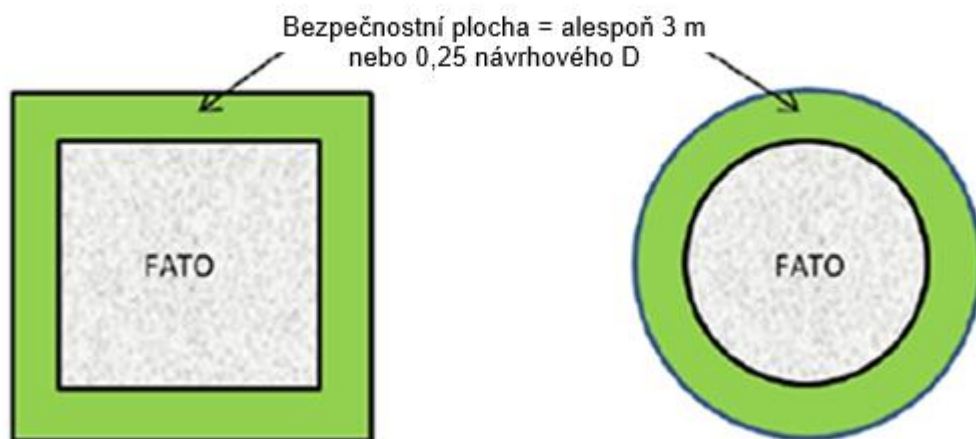
Obr. 3-1 FATO a související bezpečnostní plocha
