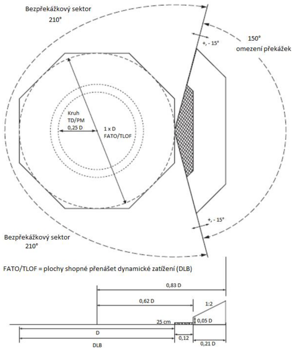
Obr. 4-83 Sektory a plochy helideku s omezením překážek pro FATO a shodný TLOF 1 D a větší.
