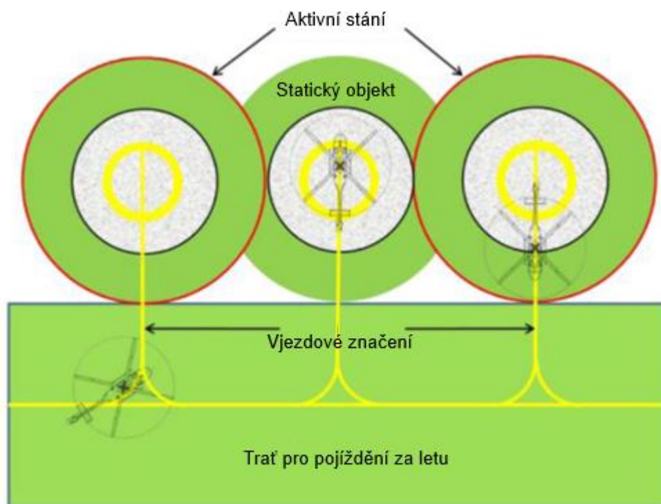
Obr. 3-8 Stání pro otáčení (s tratěmi pro poježdění za letu) – nesouběžné použití – aktivní vnější stání
