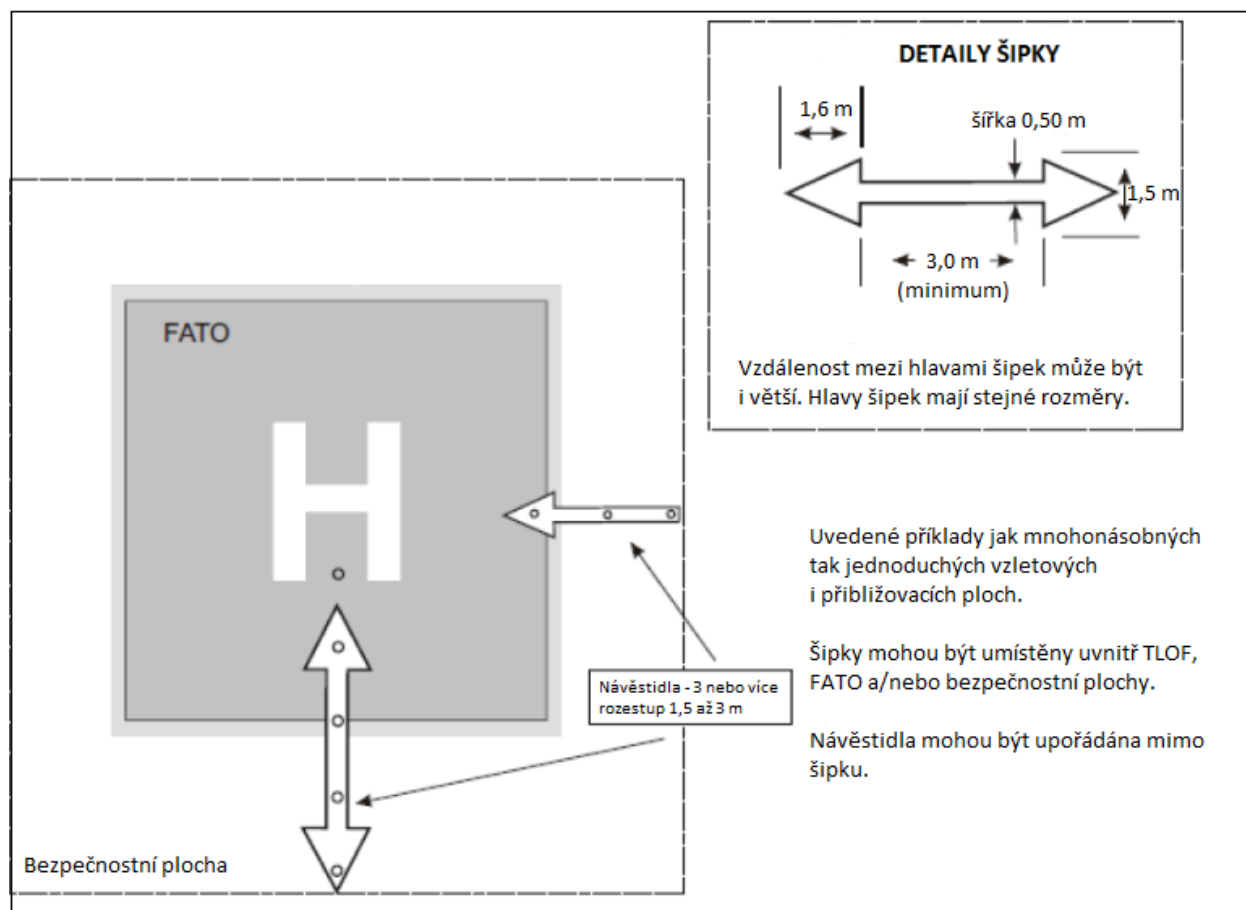
Obr. 5-109 Značení a soustava návěstidel osového vedení trajektorie letu
