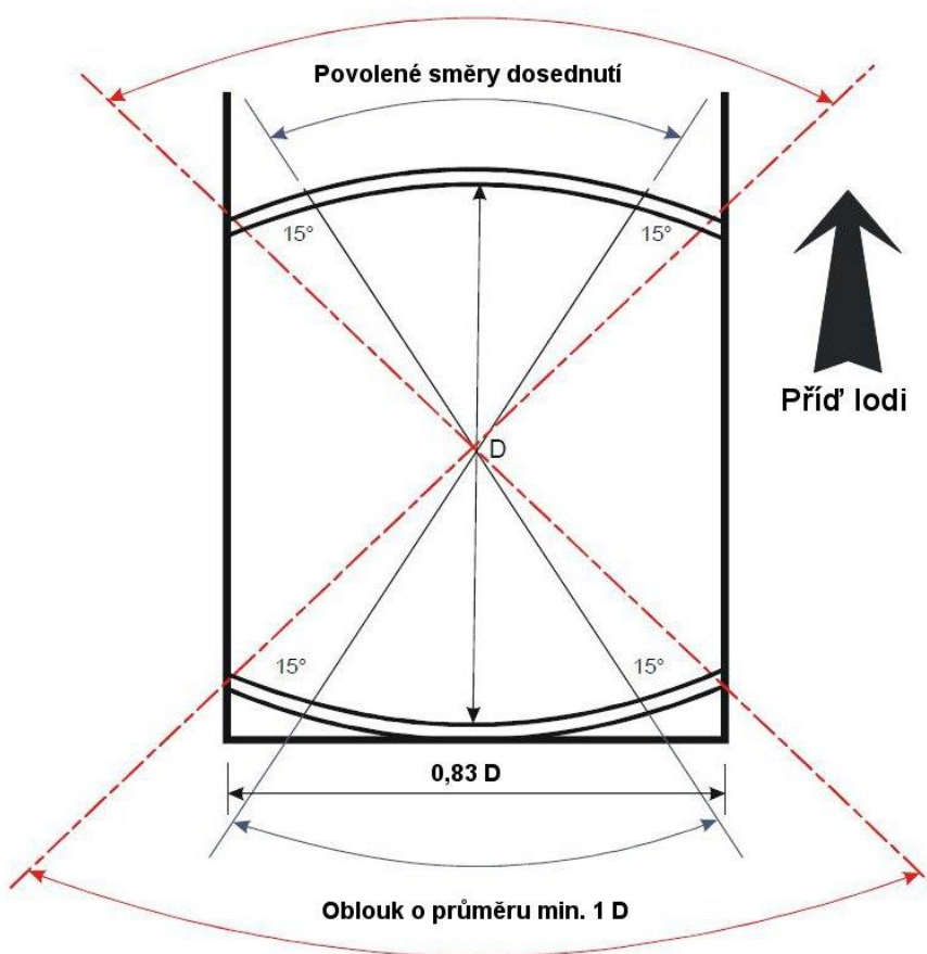
Obr. 3-107 Povolené směry dosednutí na palubách lodí během provozu se směrovým omezením.
