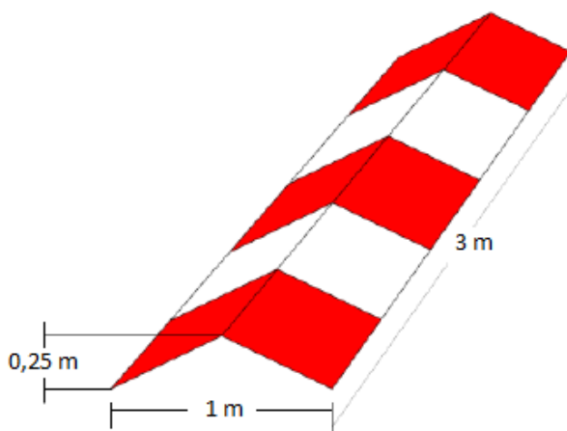
Obr. 5-65 FATO s charakteristikami RWY – postranní značka
