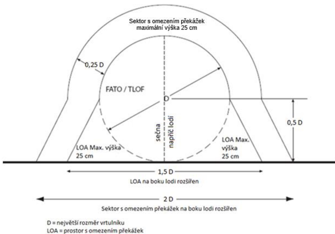
Obr. 4-146 Plochy s omezením překážek účelově vystavěného heliportu umístěného na boku lodi
