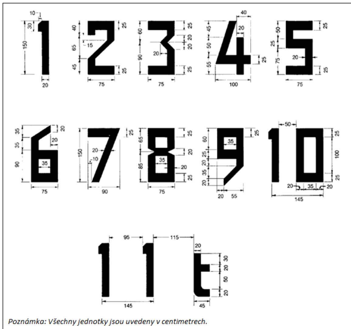
Obr. 5-54 Formát a velikost číslic a písmen
