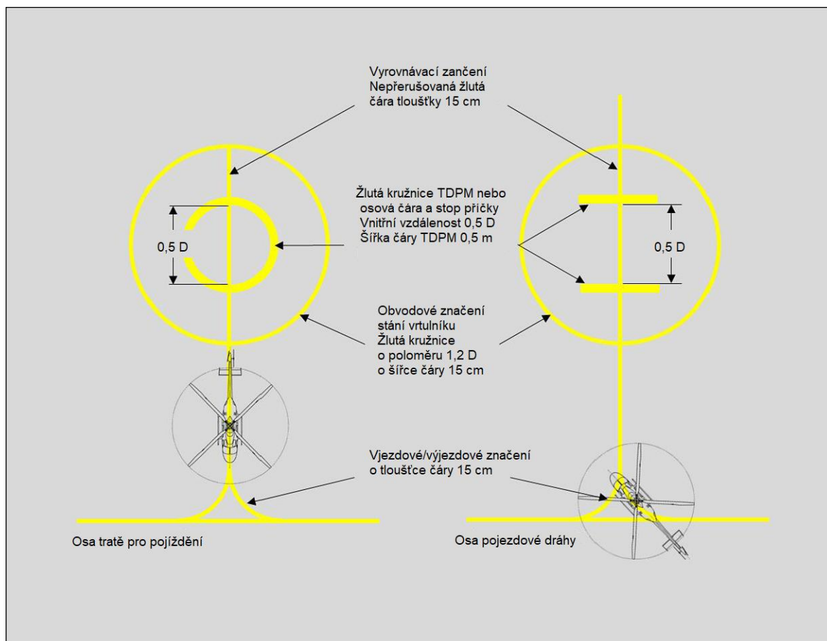
Obr. 5-98 Značení stání vrtulníku
