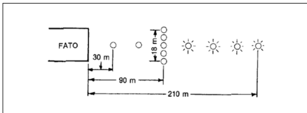
Obr. 5-132 Přibližovací světelná soustava
