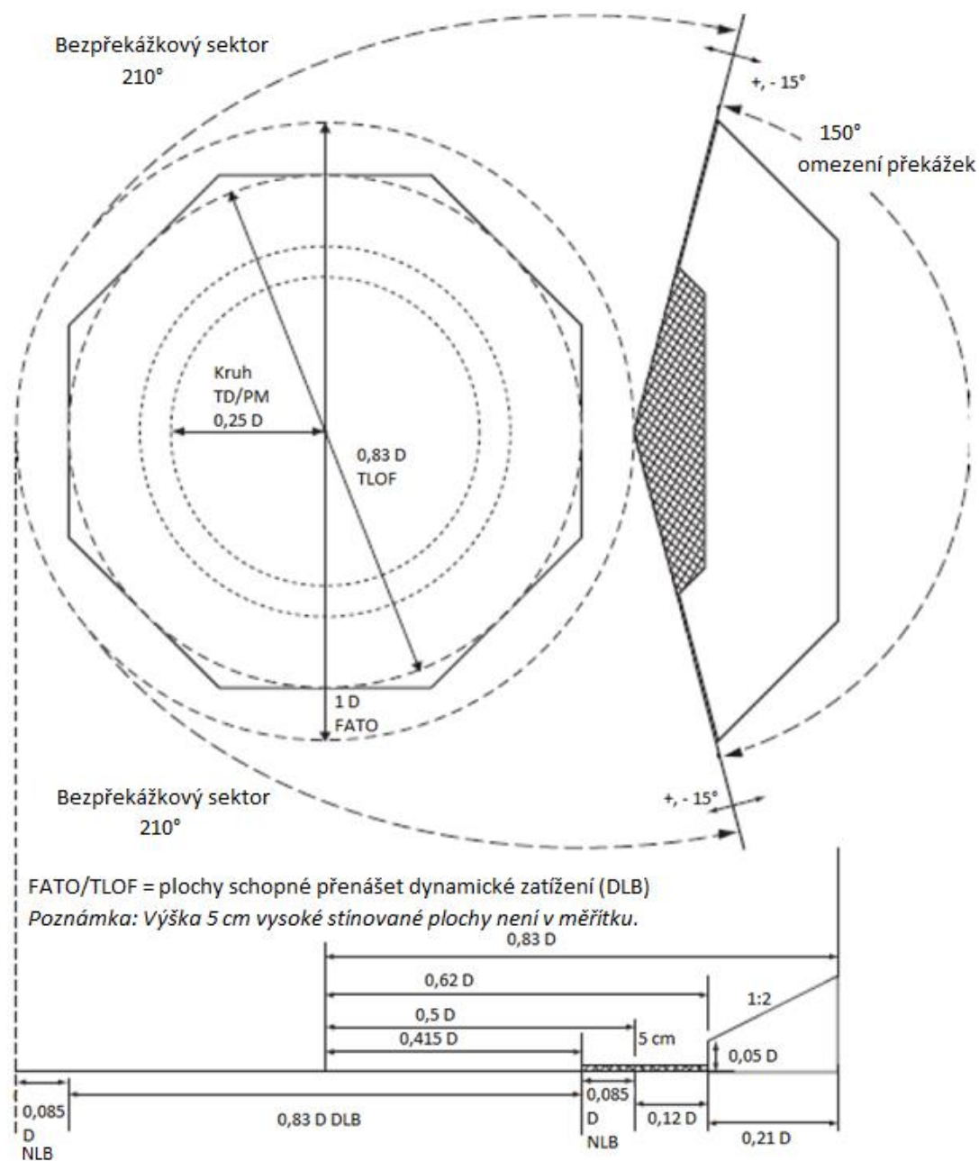
Obr. 4-94 Sektory a plochy helideku s omezením překážek pro TLOF 0,83 D a větší
