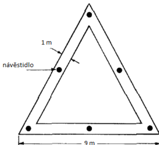
Obr. 5-76 Značení zaměřovacího bodu
