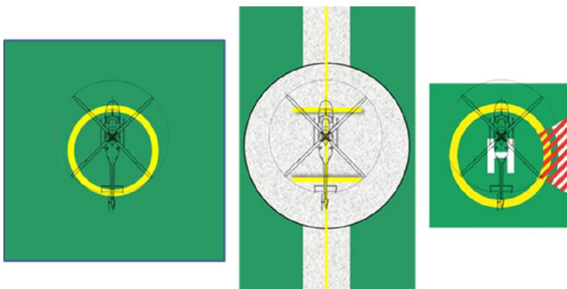
Obr. 5-87 Vícesměrový TDPC bez omezení (vlevo). Jednosměrové značení postranního pásu a související osy (uprostřed). Vícesměrový TDPC se značením sektoru se zákazem přistání (vpravo)
