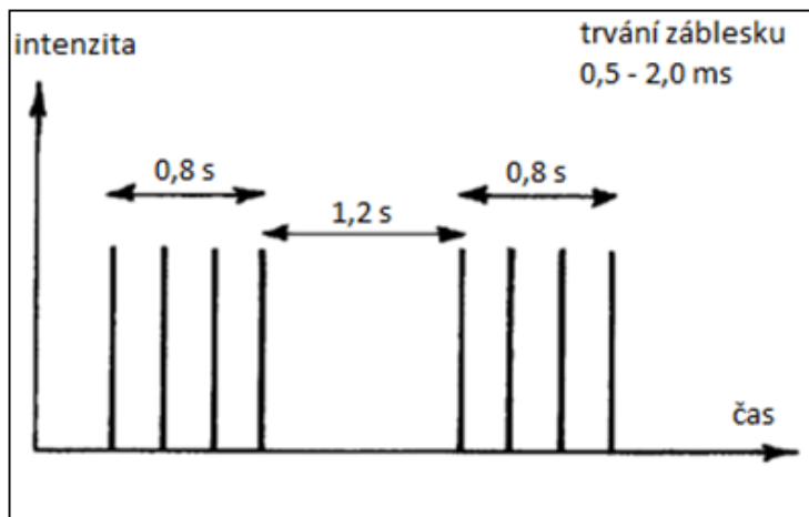
Obr. 5-110 Charakteristiky zábleskového majáku heliportu
