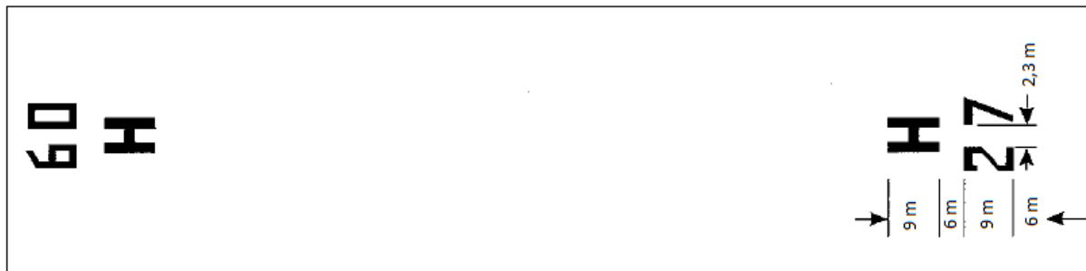
Obr. 5-3 Poznávací značení FATO a poznávací značení heliportu pro FATO s charakteristikami RWY
