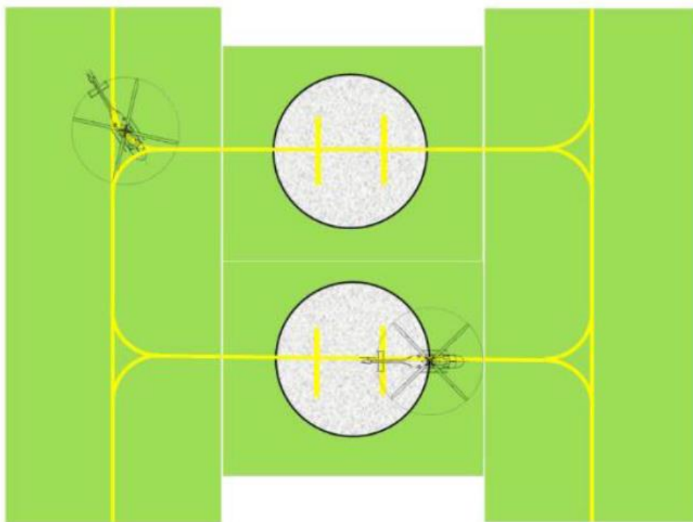
Obr. 3-7 Stání pro průjezd za letu (s tratí pro poježdění za letu) – souběžné použití
