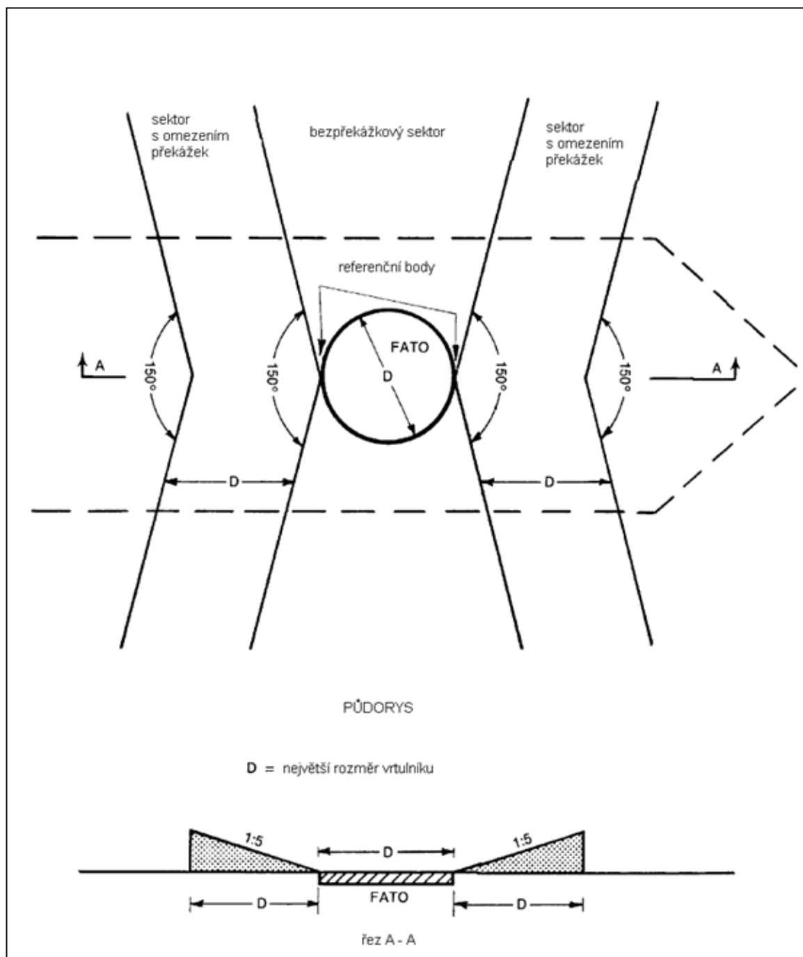
Obr. 4-105 Plochy s omezením překážek neúčelově vystavěného heliportu umístěného uprostřed lodi
