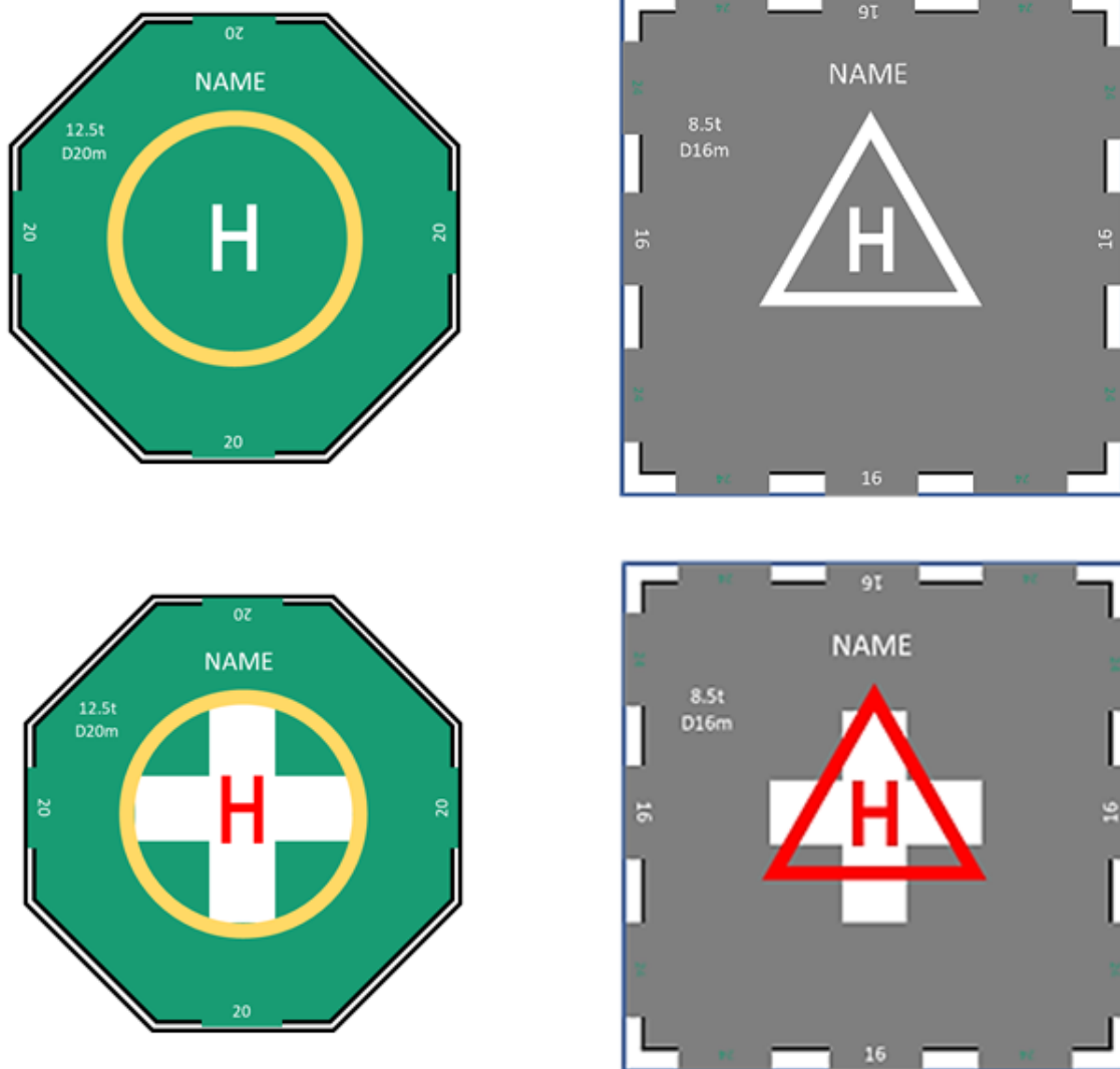
Obr. 5-1A2 Poznávací značení heliportu s TLOF a značení zaměřovacího bodu heliportů a heliportů v nemocnicích/pro leteckou záchrannou službu
