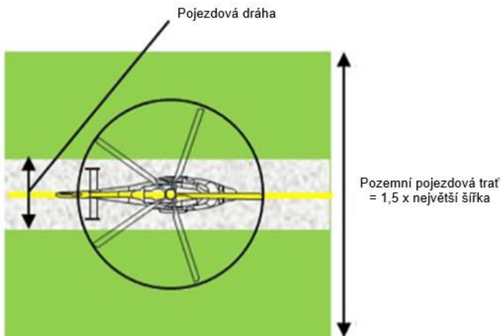
Obr. 3-3 Pojezdová dráha pro vrtulníky/pozemní pojezdová trať
